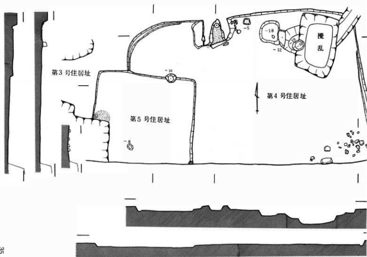
第10图 第3~5号住居址实测图 (1:80)
