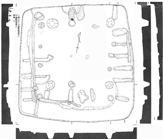
第6图 第2号住居址实测图(1:80)
