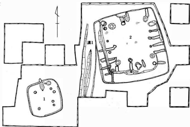
第3図 第1次調査遺構分布図(1:160)
