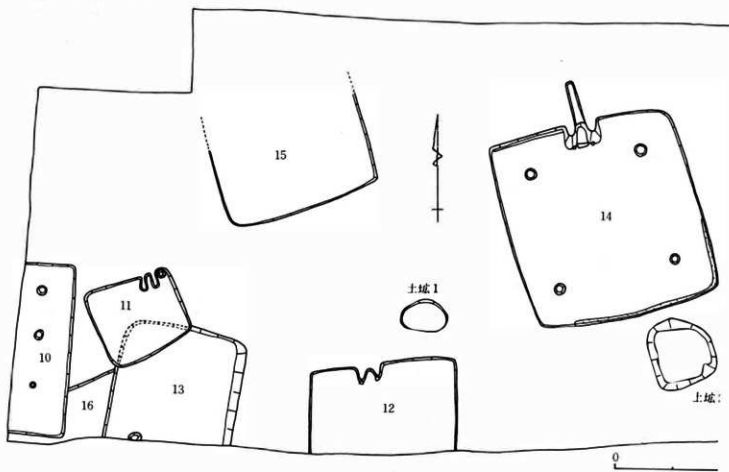
第17図 第3次調査遺構分布図 (1:160)
