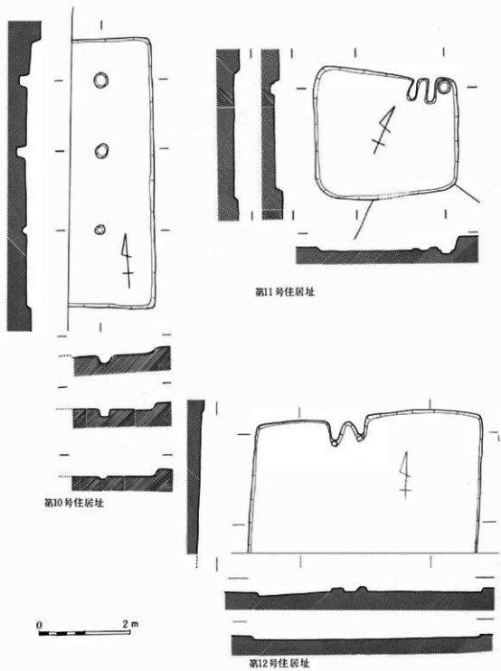
第18图 第10—12号住居址实测图 (1:80)
