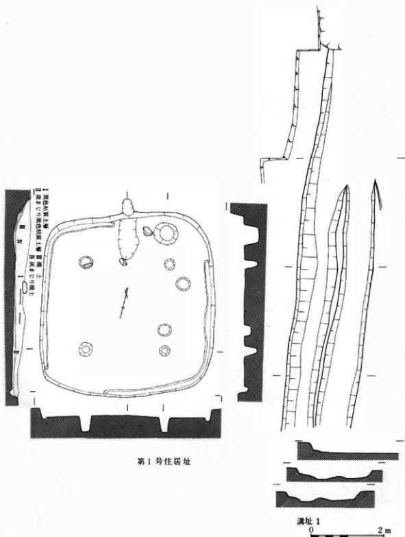
第4图 第1号住居址、沟址1实测图(1:80)
