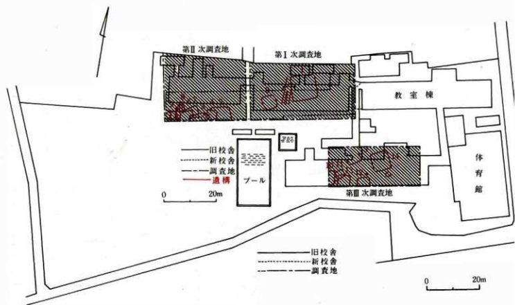
第2図 調査地及び遺構分布図 (1 : 500)
