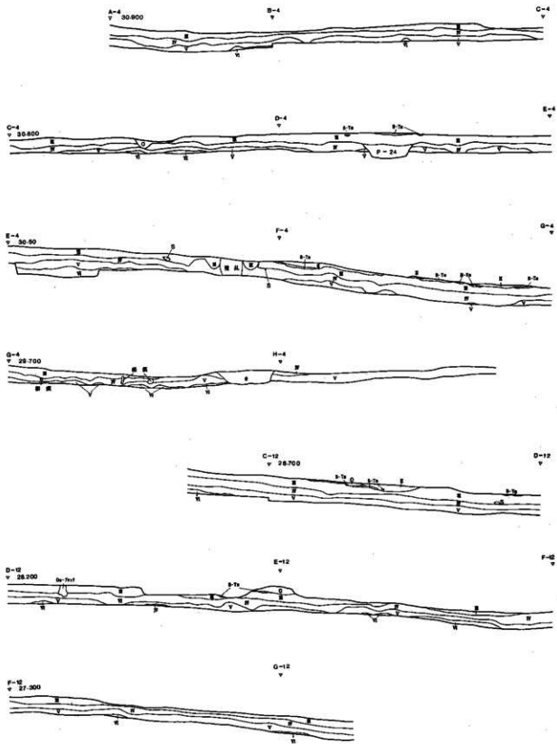
图1-8 土层断面图(3)
