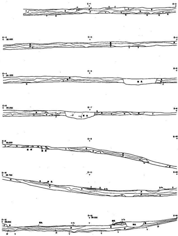
图 1-6 土层断面图(1)
