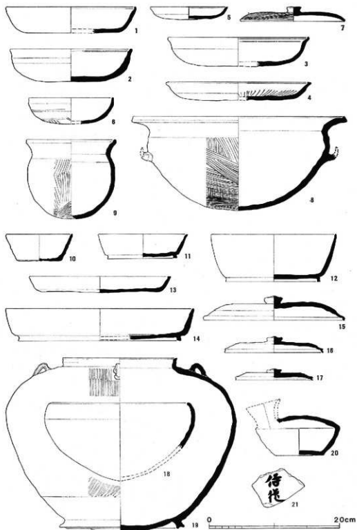
第5圖 土器実測圖
