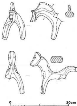
第4図 SD1545出土土馬実測図
