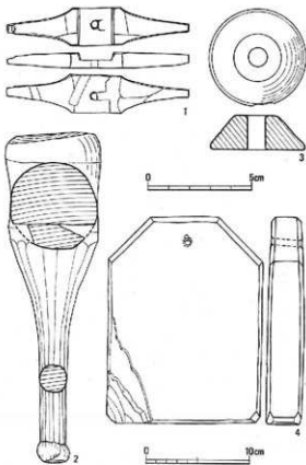
第7図 木製品・石製品実測図
