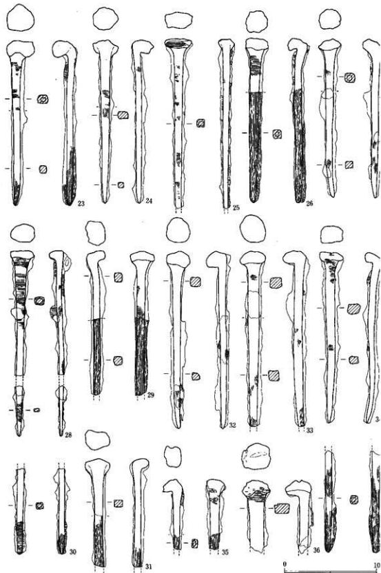
图版十六 第15支群9号墳鉄釘
