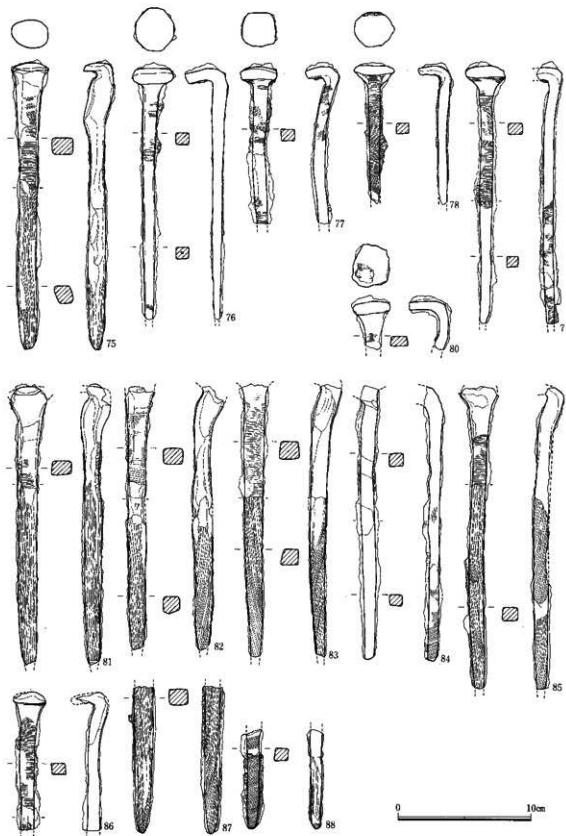
图版十八 第27支群2号墳鉄釘
