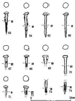
図-7 第27支群1号墳出土鉄釘
