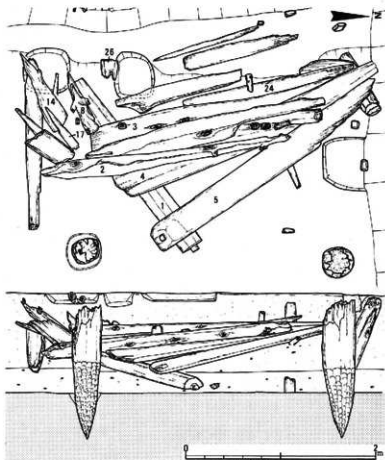
fig. 5 橋材の出土状況
