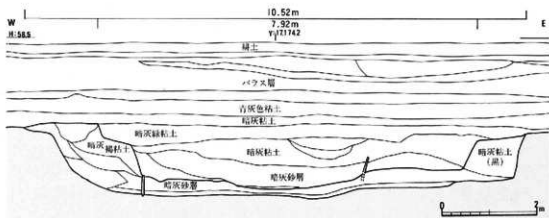
fig. 7 1975年度調査東堀河断面図
