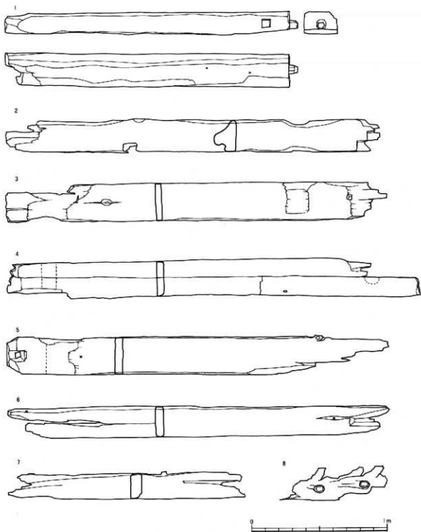
fig. 26 橋の部材
