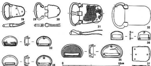
fig. 22 帯金具実測図
