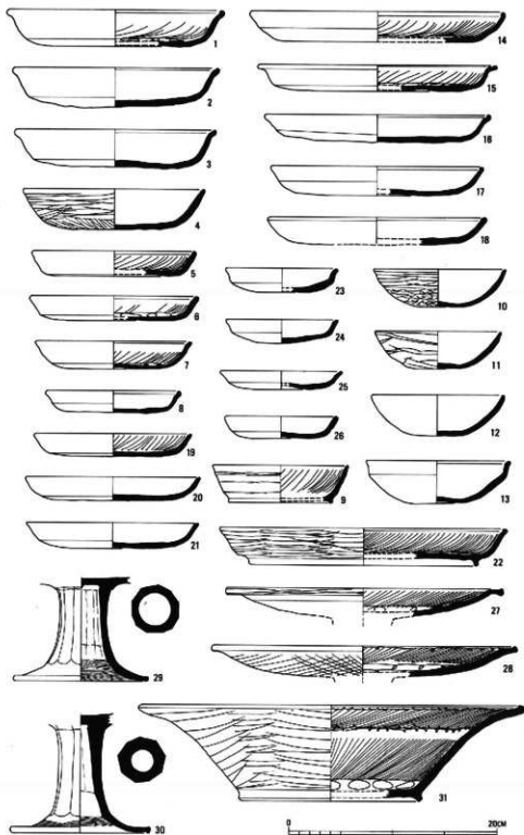
fig. 9 土師器実測図
