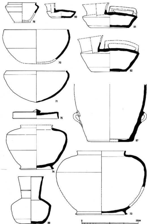
fig. 12 須惠器実測図
