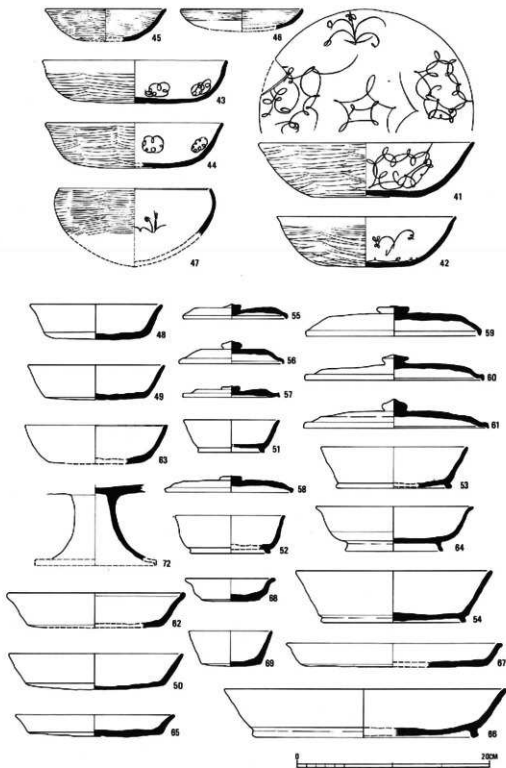
fig. 11 黑色土器·須惠器实测图
