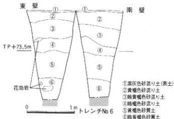
第5図 トレンチNo. 3、4、6土層断面図
