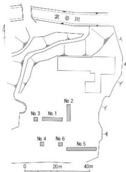
第3図 トレンチ配置図
