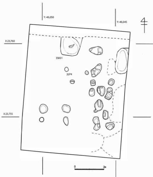
Fig.9 遺構全体図 (1/80)
