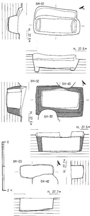
Fig. 19. SR-01~03実測図 (1/45)
