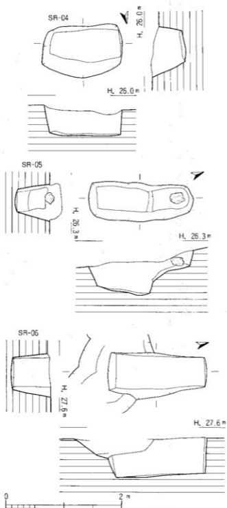
Fig. 20. SR-04~06実測図 (1/45)
