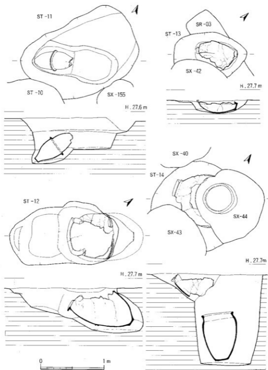
Fig. 12. ST-11~14実測図 (1/30)
