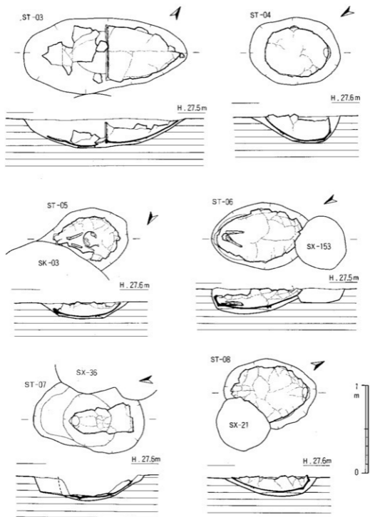
Fig. 7. ST-03~08実測図 (1/30)
