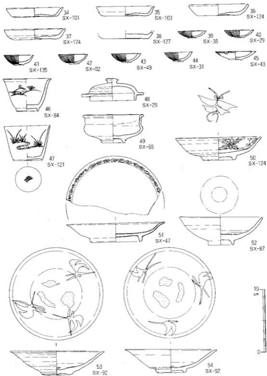
Fig. 25. 近世墓供獻土器実測図(1) (1/3)
