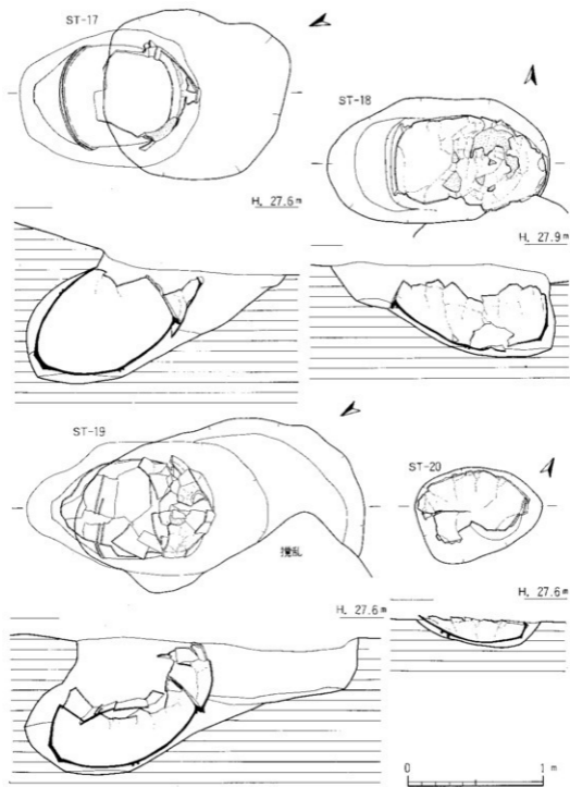
Fig. 16. ST-17~20実測図 (1/30)
