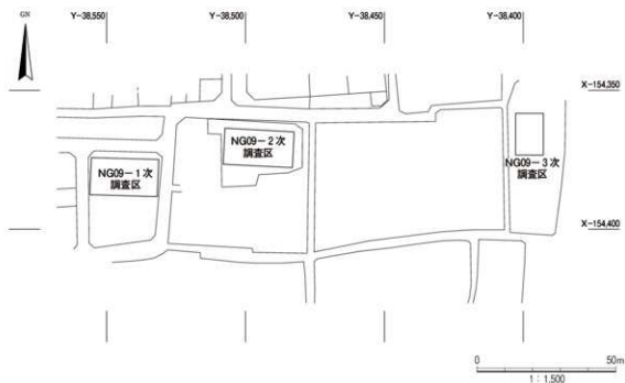
図4 調査区位置図
