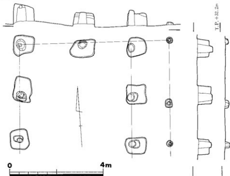
図12. 建物1 平面・断面図
