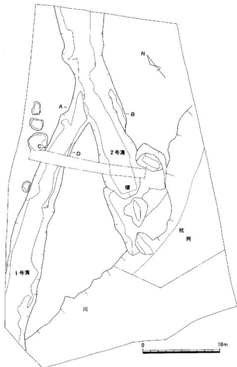
第4図 1区1・2号溝全体図 (1/250)
