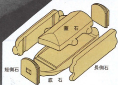
石棺展開図
