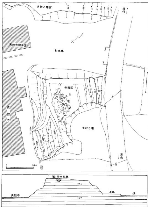
Fig. 1 地形測量図 (縮尺 1/400)
