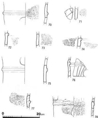
第13図 円筒埴輪 筒部「Ⅰ類・Ⅱ類」実測図(1/6)
