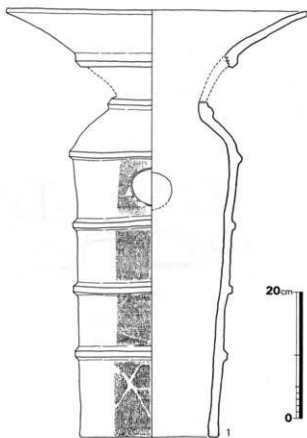
第21図 復原円筒埴輪実測図①(1/6)
