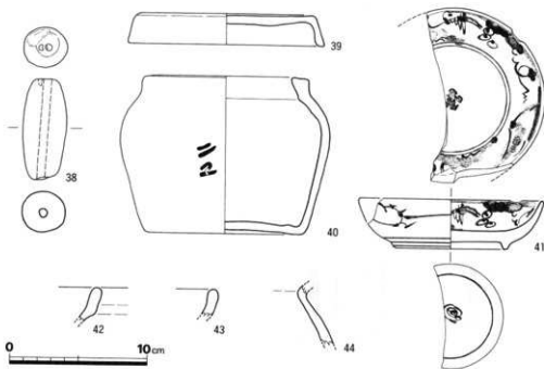
第9図 その他の遺物実測図 (1/3)
