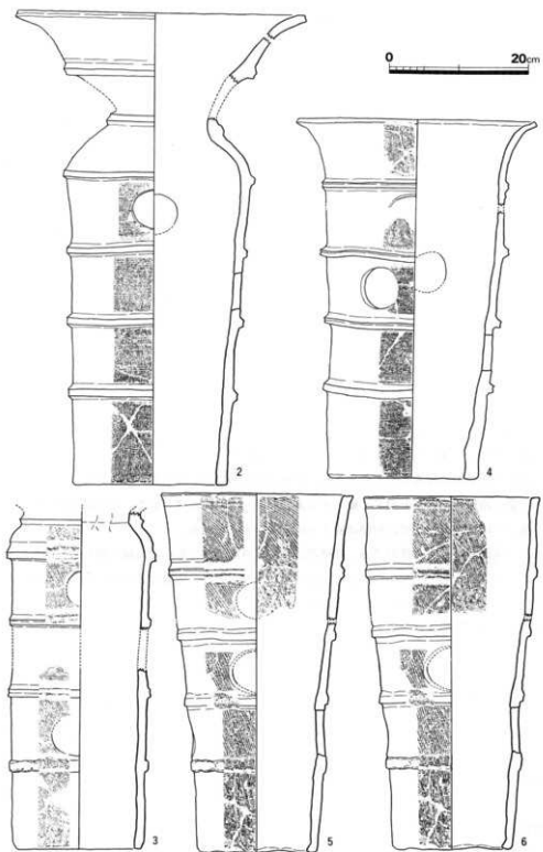
第22図 復原円筒埴輪実測図 ② (1/6)
