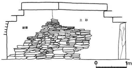
第19圖 久塚古墳石室南側壁推定復原圖
