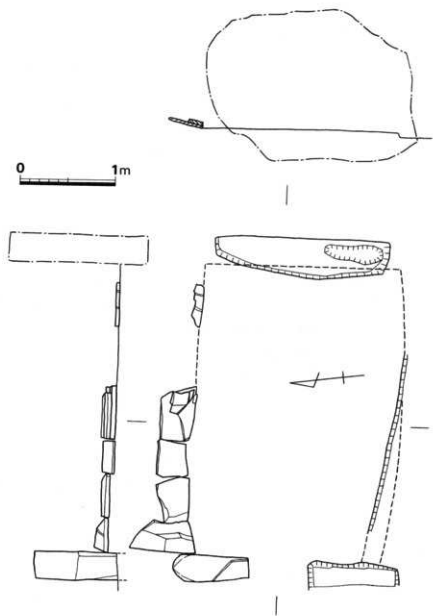
第4圖 穴塚古墳石室実測圖 (1/40)
