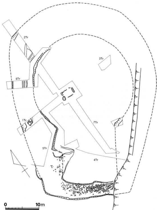
第2圖 穴塚古墳墳丘測量圖
