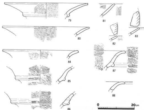
第14図 朝顔形円筒埴輪 口縁部「Ⅰ類・Ⅱ類」実測図 (1/6)
