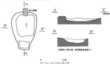
第6図 4面遺構図(鍛冶炉)
