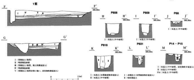
第9図 9面遺構図 (竪穴状遺構・ピット)
