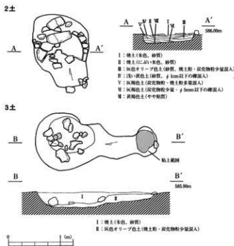
第4図 3面遺構図(鍛冶炉)
