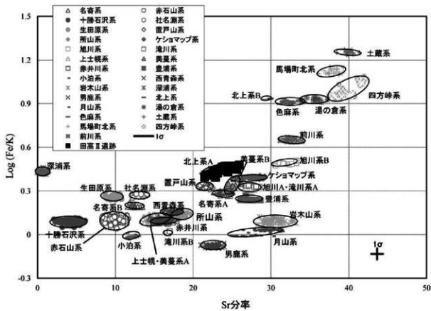
附図10 黒曜石原産地の判別図2
