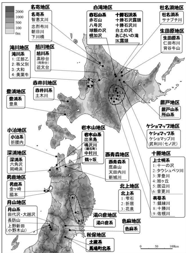
附図 11 石器時代における北海道・東北地方の黒曜石原産地
