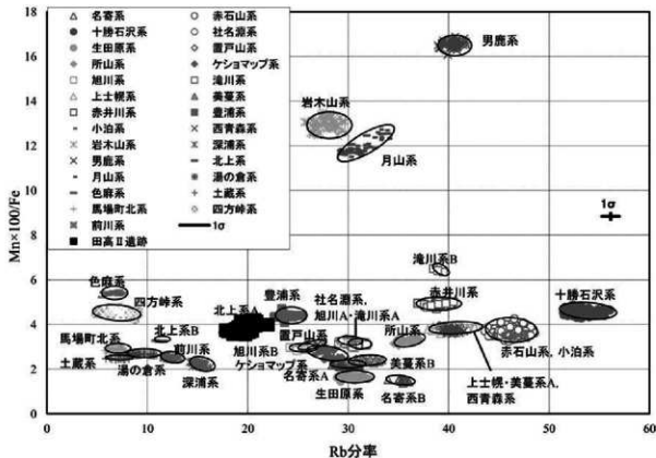
附図9 黒曜石原産地の判別図1
