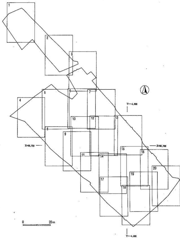
図版1 割付図の配置 1 : 800
