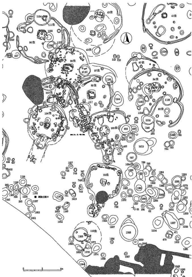
図版10 遺構新付図(9) 1 : 120
