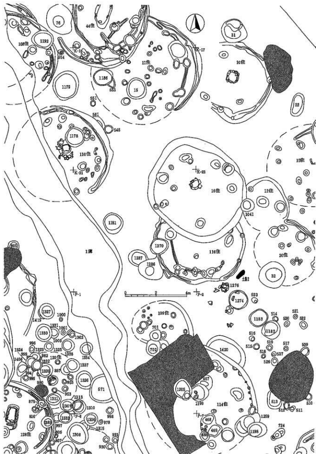
図版16 遺構制村図04 1 : 120
