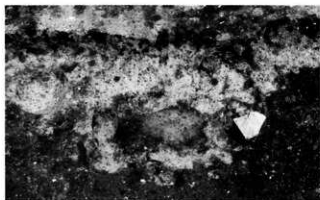
②H9号住居址カマド
