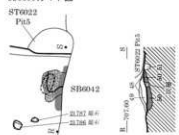
SB6069カマド図
