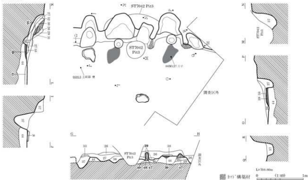
カマドの構造材 0 (1:400) 2m
