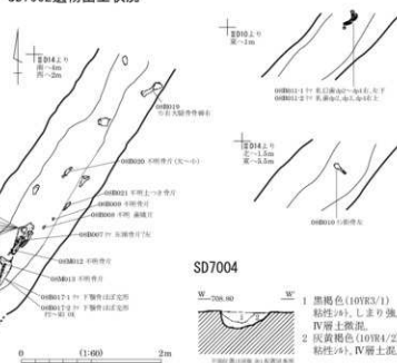
SD7002遺物出土状況
