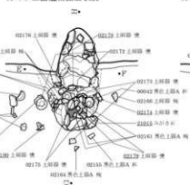
SB0073 カマド上面遺物出土状況
