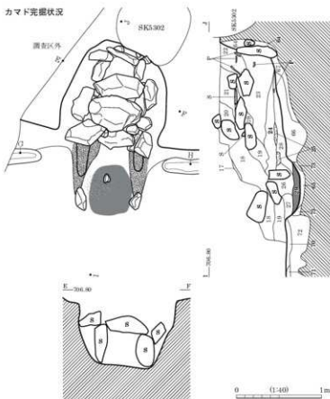
カマド完備状況
