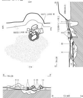
SB0098 カマド図
