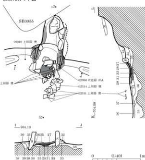
SB0078カマド図
