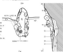
SB0073 カマド下面遺物出土状況
