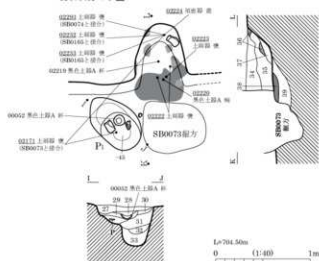
SB0164カマド図
