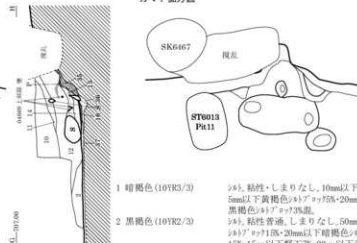
カマド断面図
