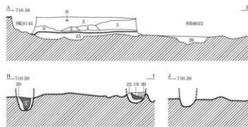
カマド遺物出土状況
