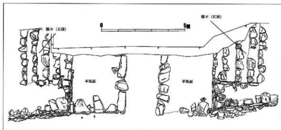
広小路御舟入石垣実測図
