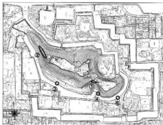
彦根城跡石垣保存修理箇所位置図
