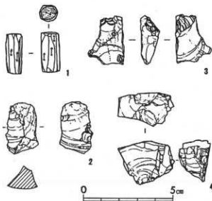
図12 高広遺跡Ⅱ区出土碧玉製管玉未成品実測図 (『高広遺跡』1984より)
