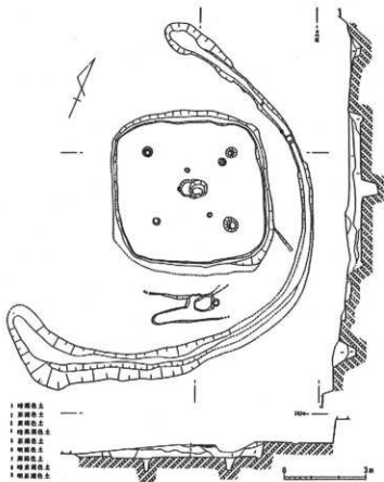
図19 平所遺跡の玉作工房跡 （『国道9号バイパス予定地内調査報告書』II 1977より）
