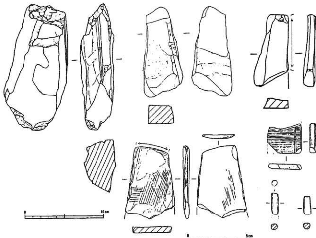
図16 布田遺跡出土の玉類未成品(碧玉製作工程) (「国道9号バイパス予定地内調査報告書」IV 1983より)
