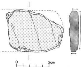
図112 又下遺跡出土の内磨砥石
