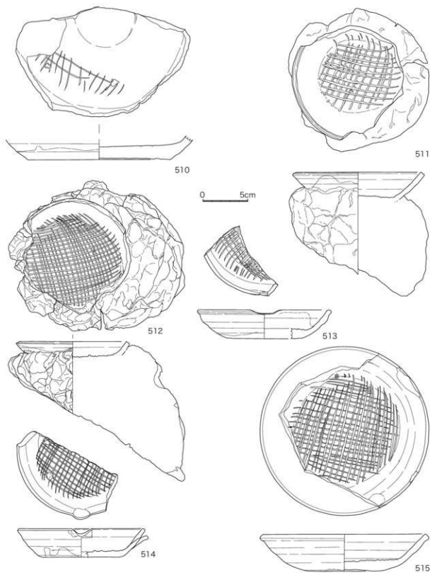
图48 灰原上層出土遺物4(1:3)
