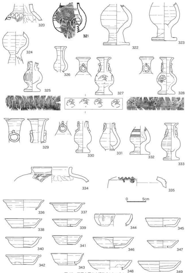
图 40 灰原中層出土遺物 8 (1 : 3)
