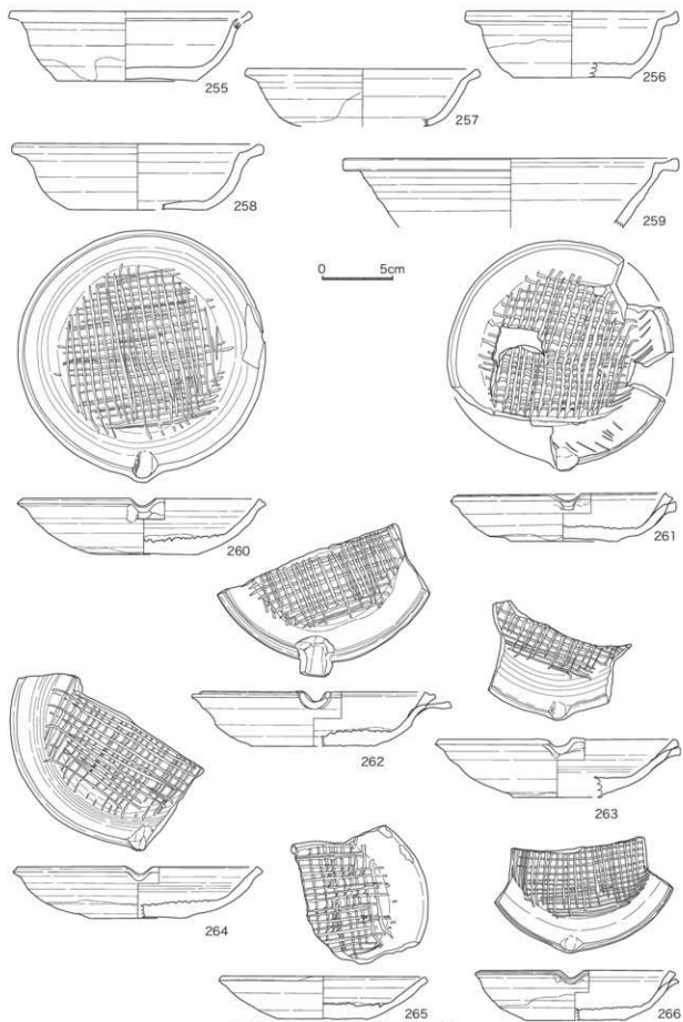
图 35 灰原中層出土遺物 3 (1 : 3)
