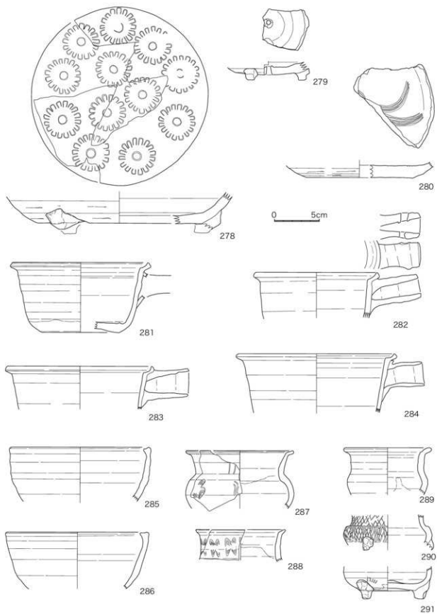
图 37 灰原中層出土遺物 5 (1 : 3)
