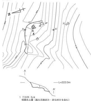
図26 SK06・SK07(1:40)
