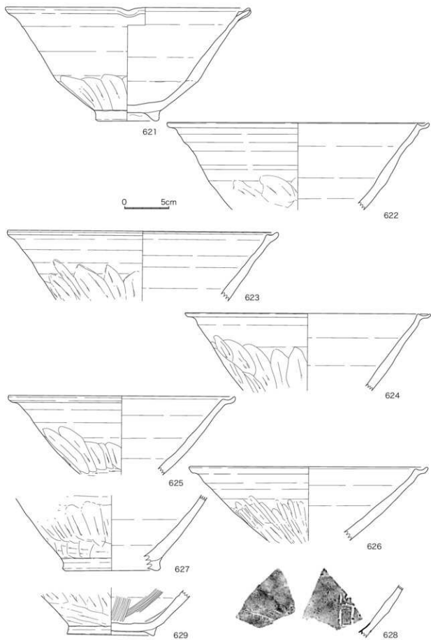
图 54 灰原上層出土遺物 10(1 : 3)
