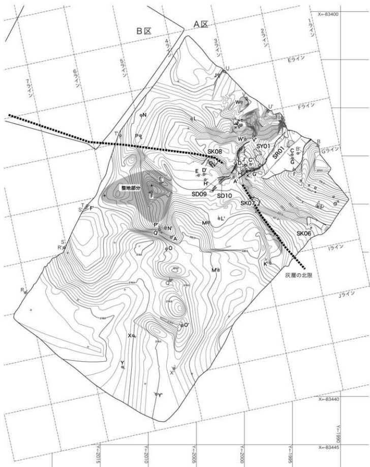
図 23 築構時遺構配置図 (1 : 200)
