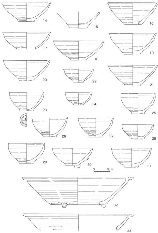
図 12 宇トグ案跡出土遺物2(1:3)
