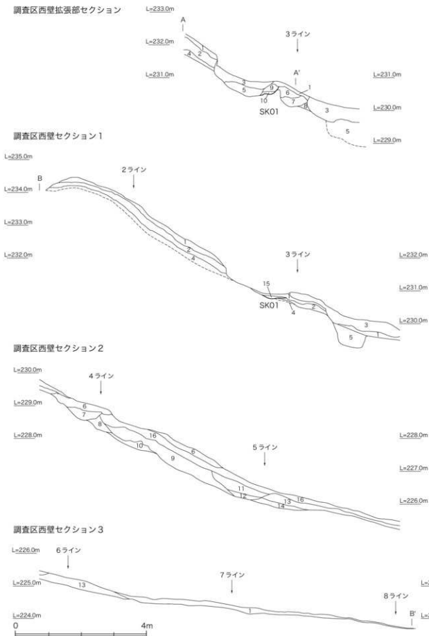
図7 灰層セクション図1 (1 : 80)
