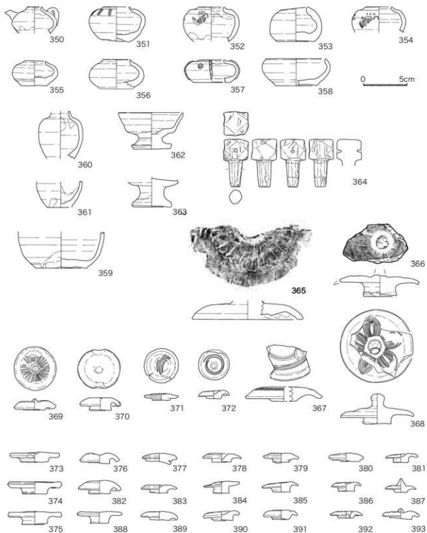
图41 灰原中層出土遺物9(1:3)
