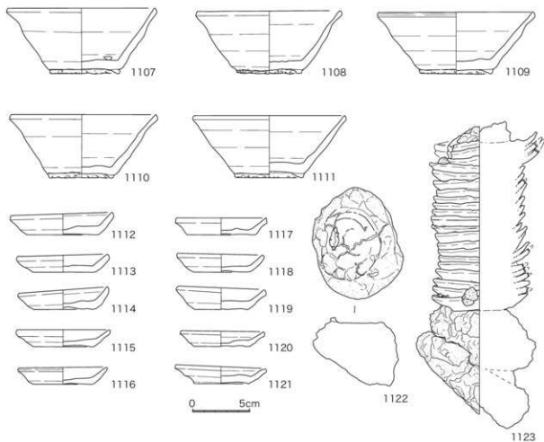
図 77 海上B窯跡出土遺物(1:3)
