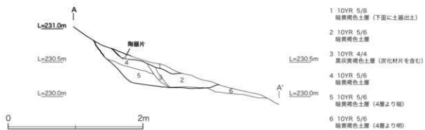
図 10 SK01(1 : 40)
