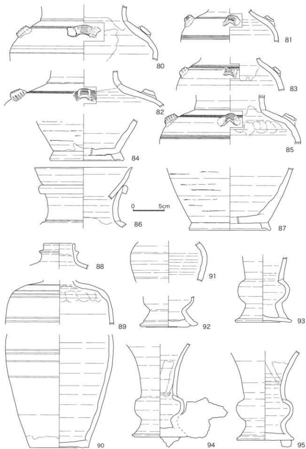
図 17 宇トグ案跡出土遺物 7(1:3)
