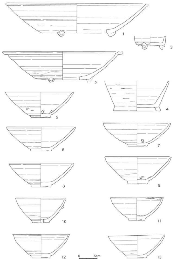
図 11 宇トク窯跡出土遺物 1 ( 1 : 3 )
