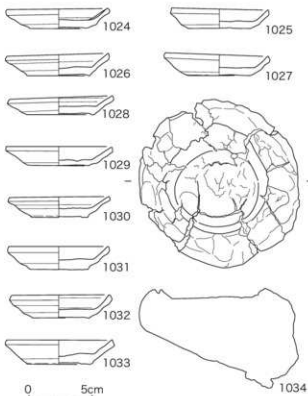
図73 広久手第26号窟跡出土遺物2(1:3)
