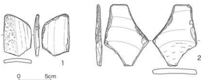
図70 黒笹40号窯跡出土陶器片転用「調整具」(1:3)
