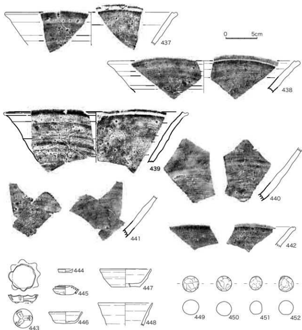
図44 灰原中層出土遺物 12(1:3)
