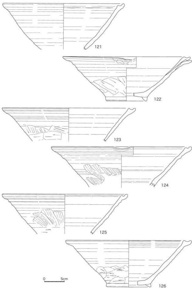
図 19 宇トグ窯跡出土遺物9(1:3)
