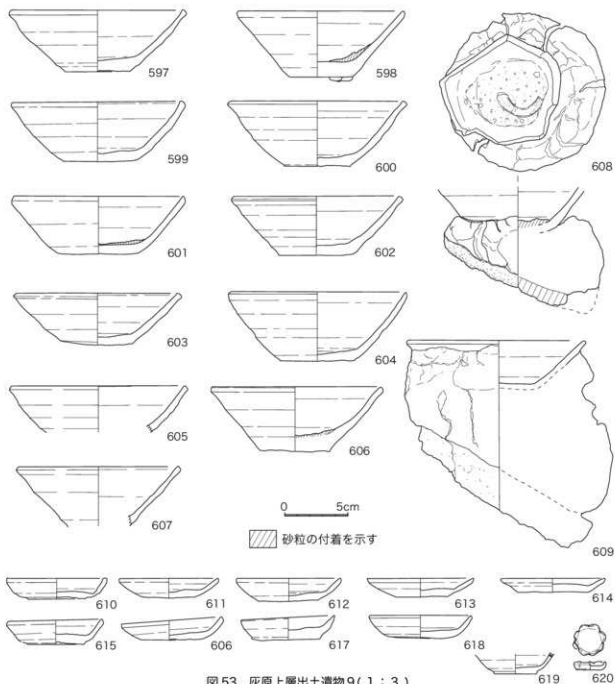
図 53 灰原上層出土遺物9(1:3)
