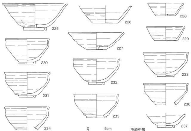
圖33 SK06・08、灰原下層、灰原中層出土遺物1(1:3)
