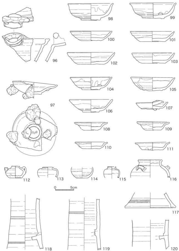
図18 宇トグ窯跡出土遺物8(1:3)
