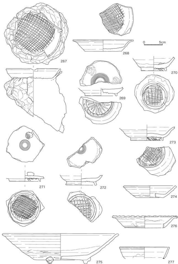
图36 灰原中層出土遺物4(1:3)
