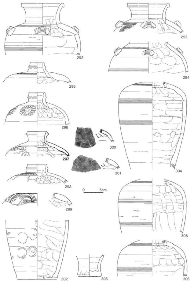
图 38 灰原中層出土遺物 6 (1 : 3)
