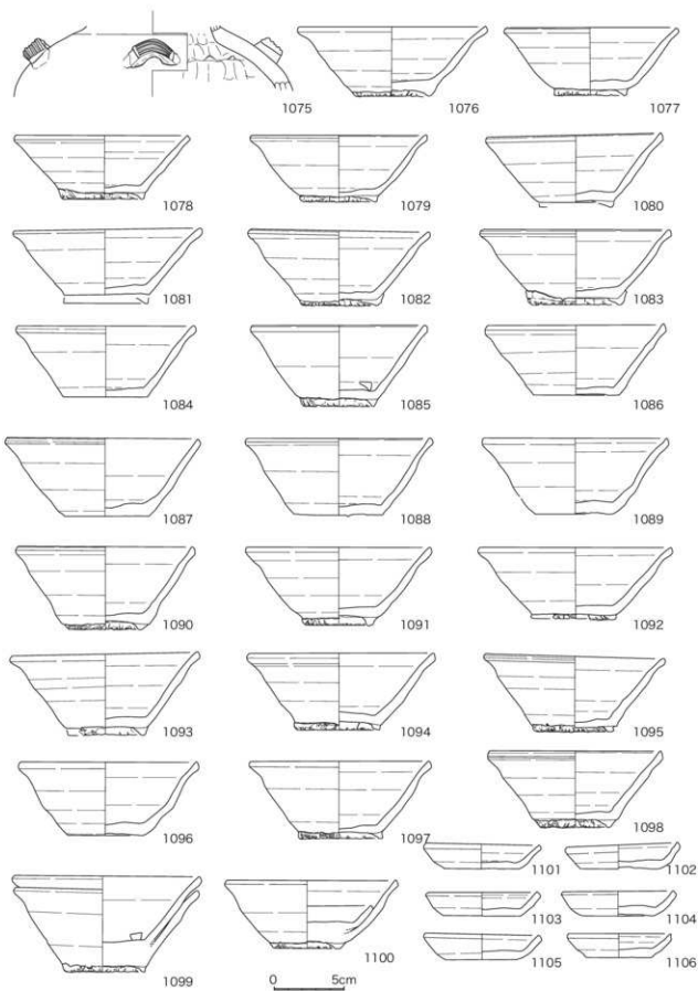
图 76 广久手第 27 号窯跡出土遺物 (1 : 3)
