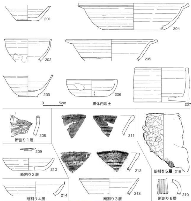
図 32 SY01 出土遺物 (1 : 3)
