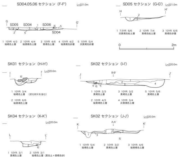
図 61 中洞窟跡B区遺構埋土セクション(1:80)
