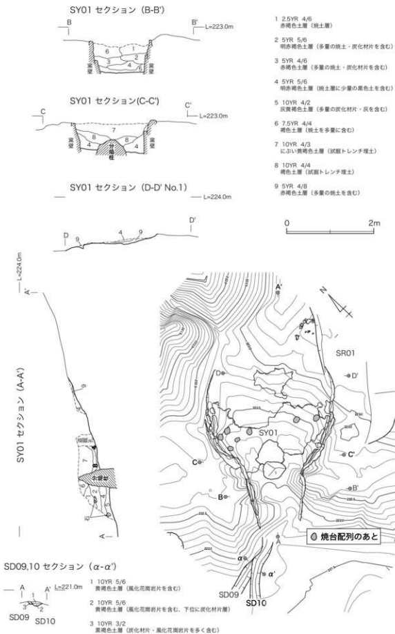
図 24 SY01・SD09・SD10 埋土堆積状況 (1:60)
