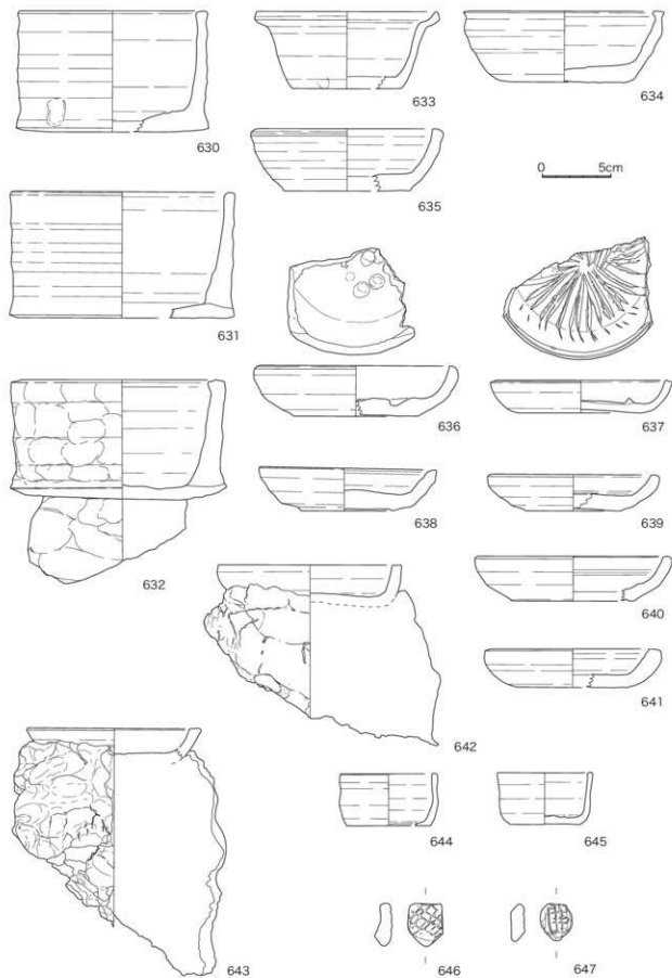
圖 55 灰原上層出土遺物 11(1:3)
