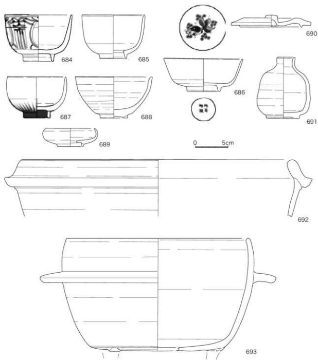
图 63 近世以降遺物実測図 (1 : 3)
