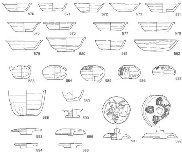
圖 52 灰原上層出土遺物 8 ( 1 : 3 )
