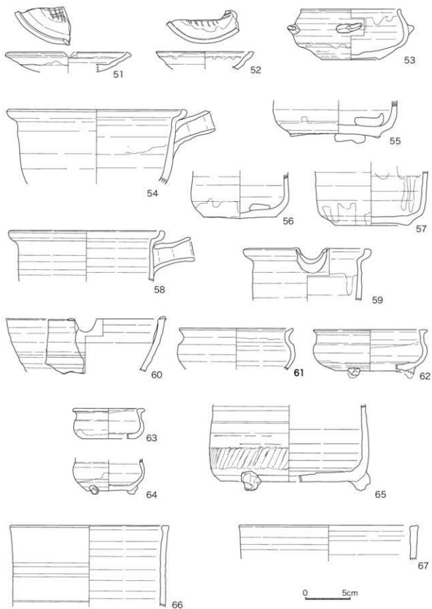
図 15 宇トグ窯跡出土遺物5(1 : 3)
