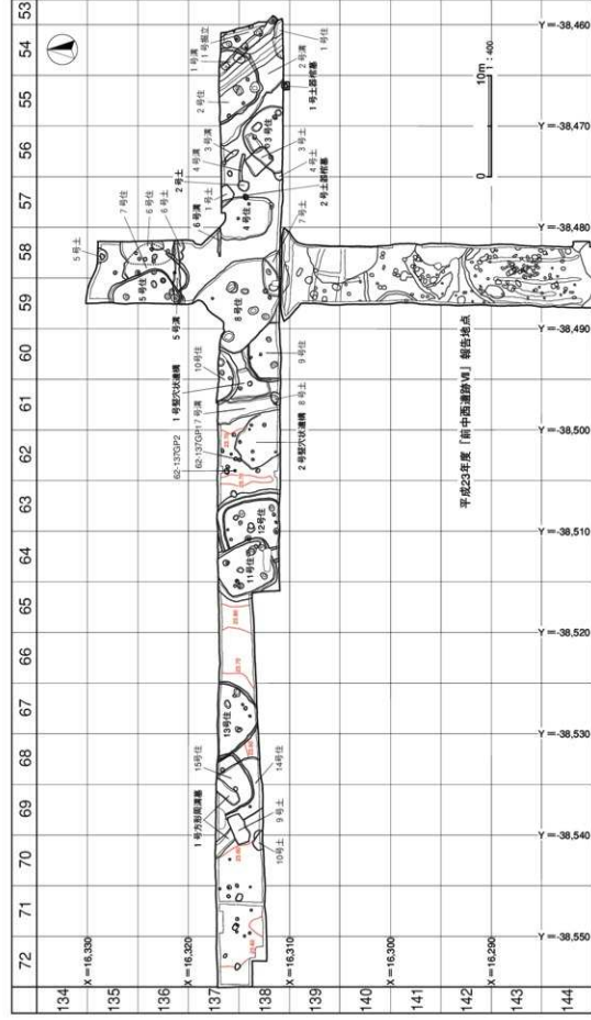
第4图 勘察区平面图
