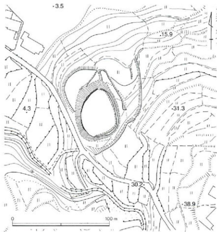
太田和氏館跡縄張り図
