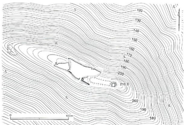
小富士城跡縄張図
