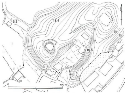
大刀洗城跡縄張図
