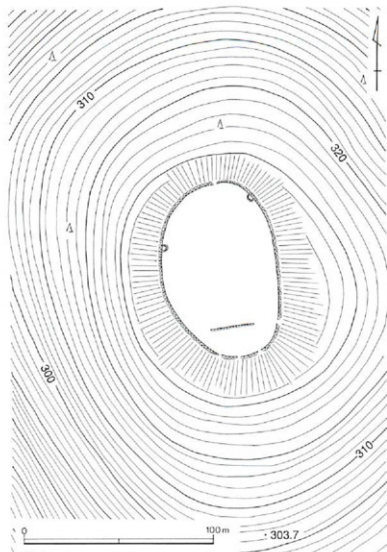
武留路山城跡縄張図
