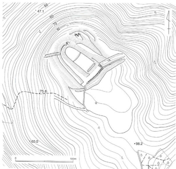
風南城跡縄張図
