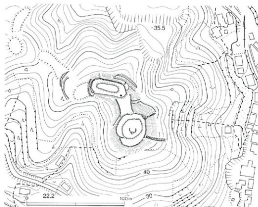
殿山城跡縮張図
