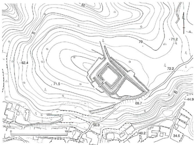
田城跡縄張図
