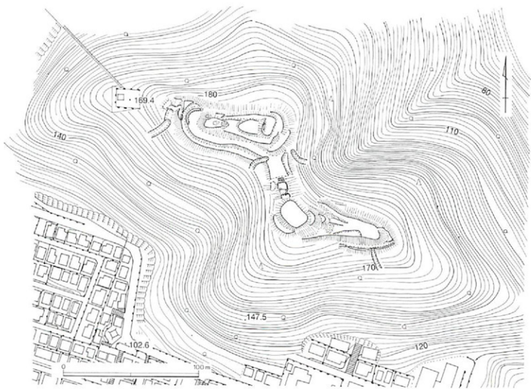
鳥山城跡縄張り図
