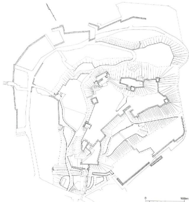
亀岡城跡縄張り図 (1/3000)
