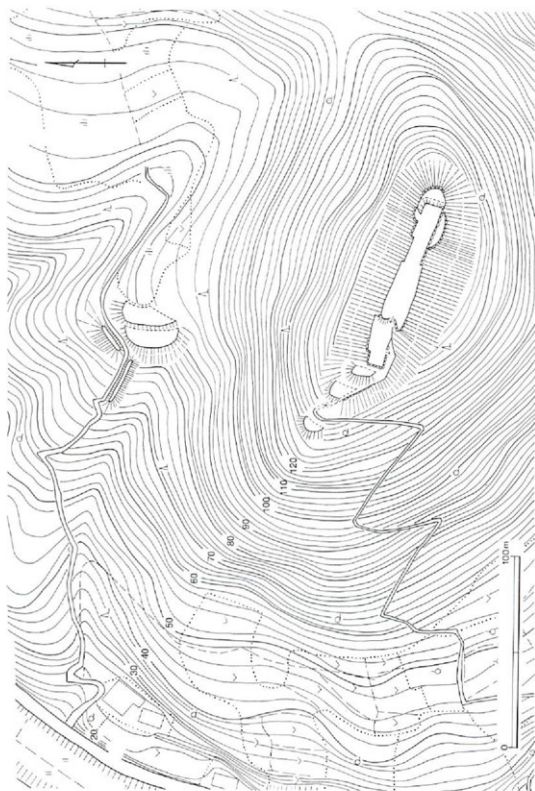
小峰城跡縄張り図
