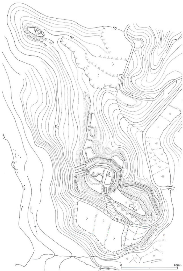
医王城跡縄張り図
