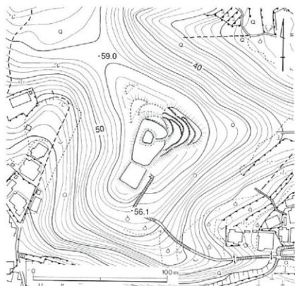
福田城跡縄張図
