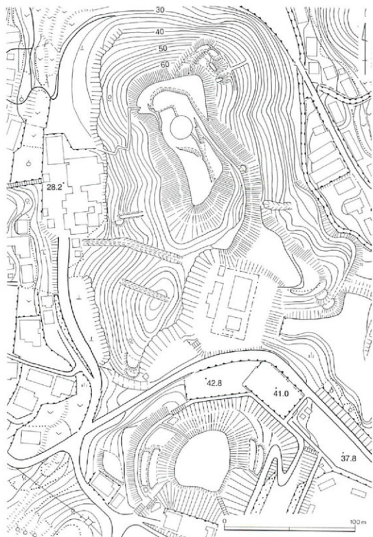
東光寺山城跡縄張り図
