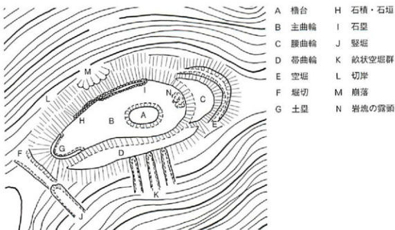
縄張図模式図
