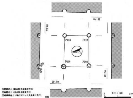
第55図 SB8・SB9
