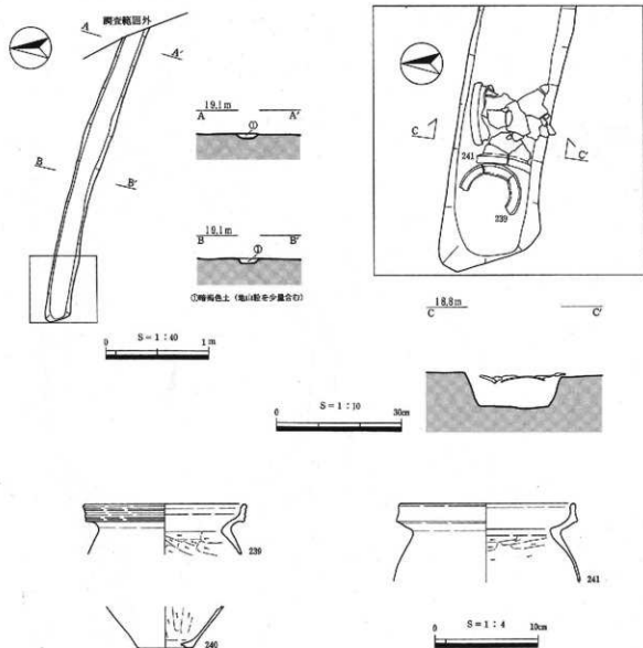
第64図 SD 5及び出土遺物
