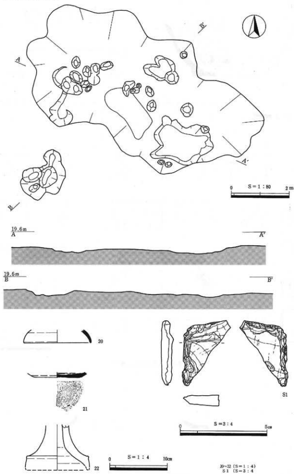
第25図 S X 1 及び出土遺物
