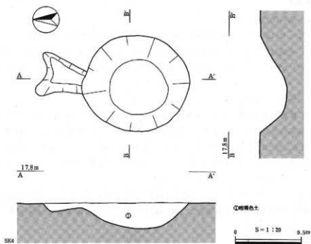
第62図 SK5・SK6
