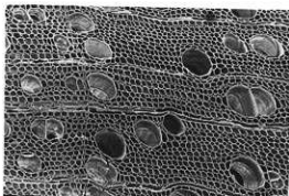
写真 7 1342 15kV x200 200 \mu m
