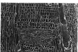
写真 11 1352 15kV x100 500 \mu m
