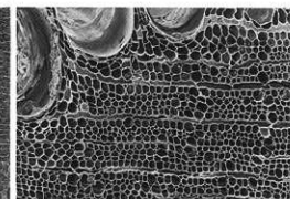
写真 20 1358 15kV x200 200μm
