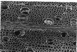
写真 10 1349 15kV x150 200 \mu m
