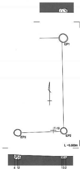
第409図 SA1002 平・断面図
