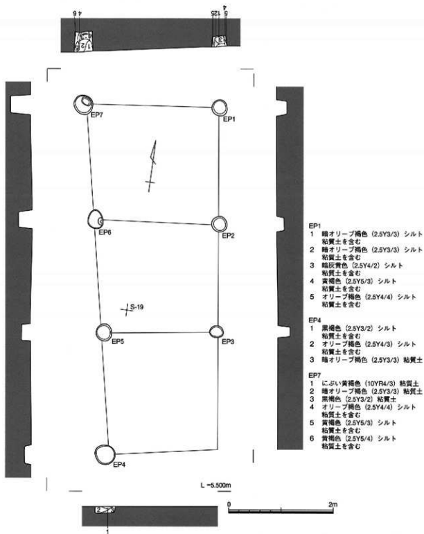
第407図 SA1001 平・断面図
