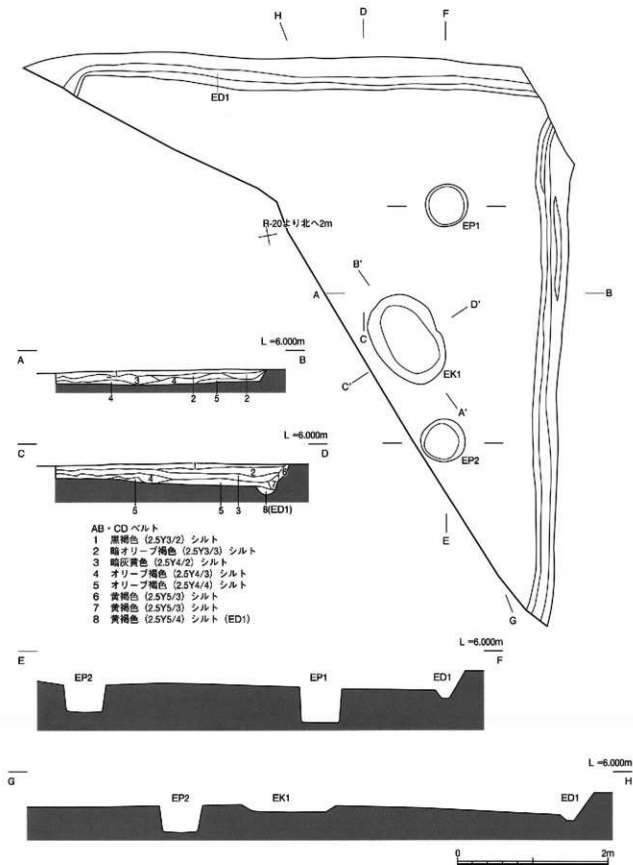
第413図 SB1001 平・断面図
