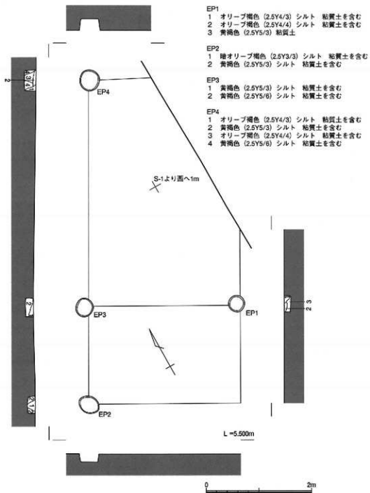
第411図 SA1003 平・断面図
