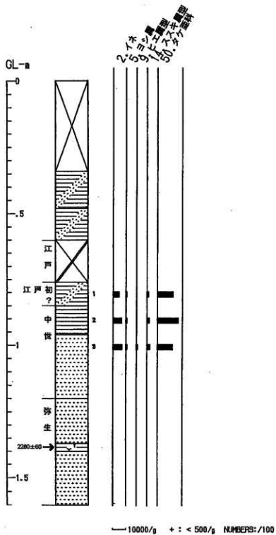
第24図 プラント・オパールダイアグラム
