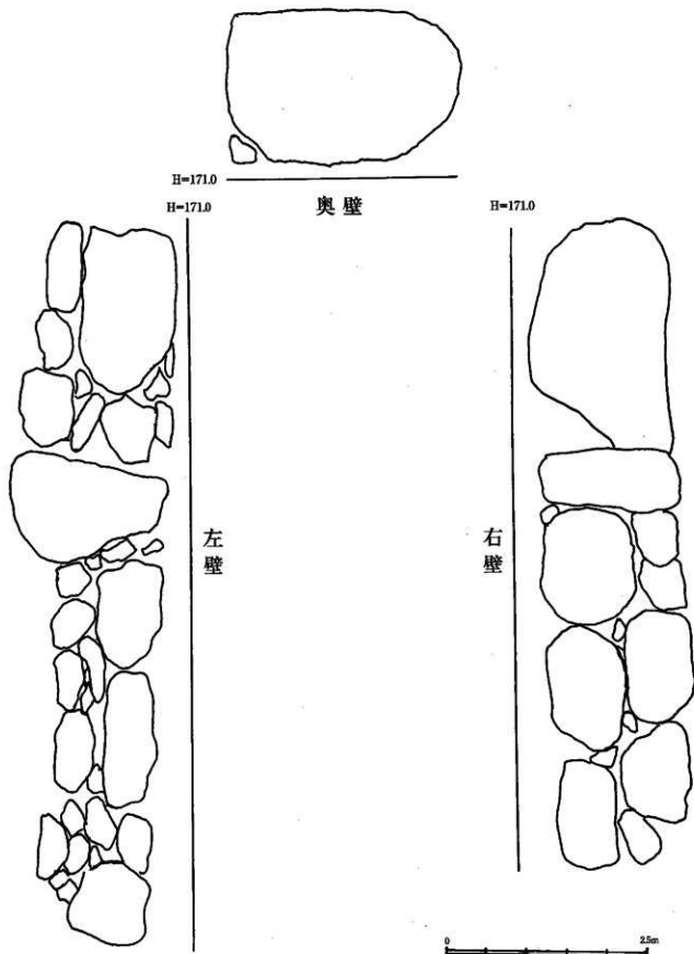
挿図2 北山2号墳石組図
