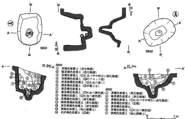
図11 SK01・02遺構図
