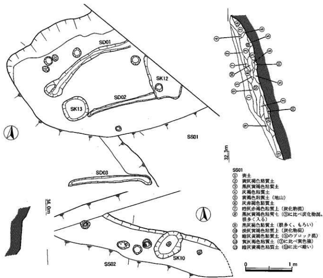
図16 SS01・02遺構図
