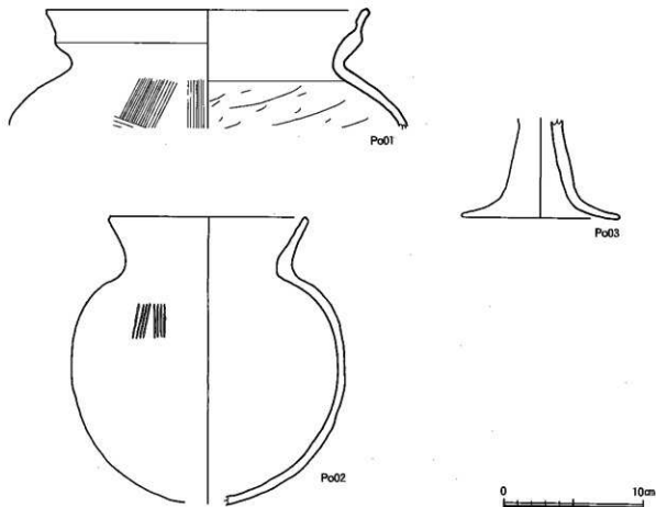
図4 S I 01出土遺物
