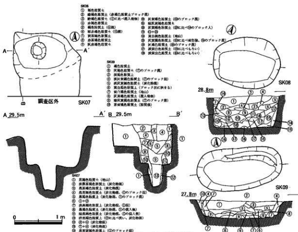
図13 SK07・08・09遺構図
