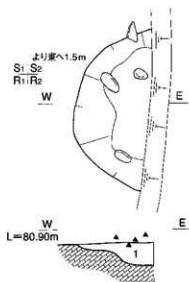
第394図 SK1010平断面図
