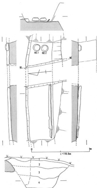
第9図 茶山1号墳第4主体図 (S=1:40)
