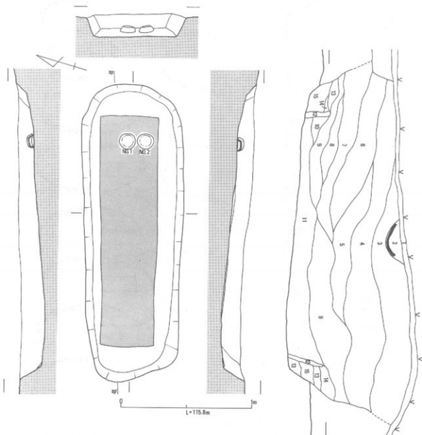
第10図 茶山1号墳第5主体図 (S = 1 : 40)
