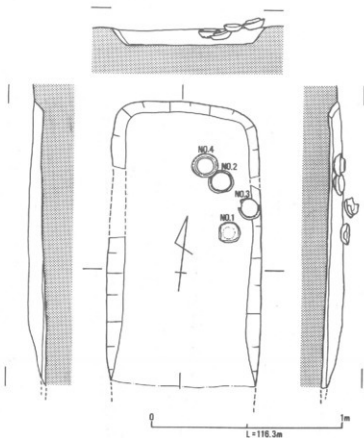
第8図 茶山1号墳第3主体図 (S=1:40)
