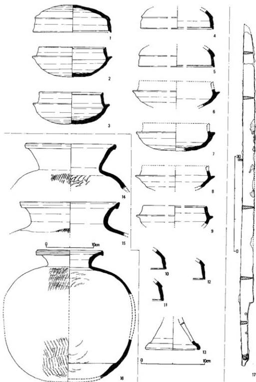
第12图 茶山1号墳出土遺物 (1~13; S=1: 3, 14~16; S=1: 4, 17; S=1: 8)
