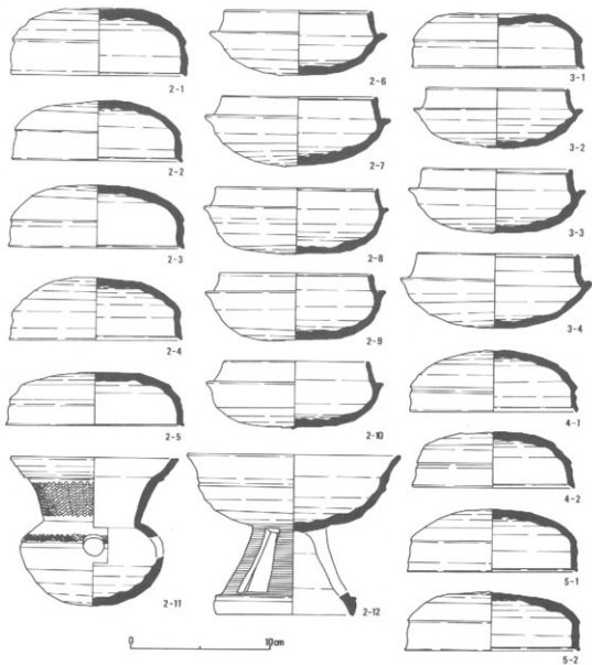
第11図 茶山1号墳2～5主体出土土器(S=1:3)
