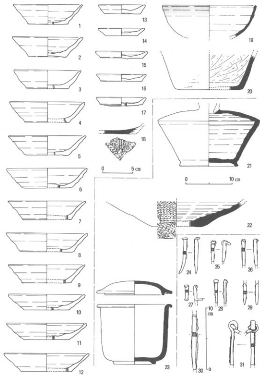
第17図 中世以降の遺物 (1~20・24~31; S=1:3、21~23; S=1:4)
