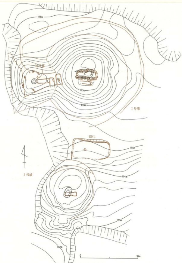
第3图 茶山古墳群地形測量图
