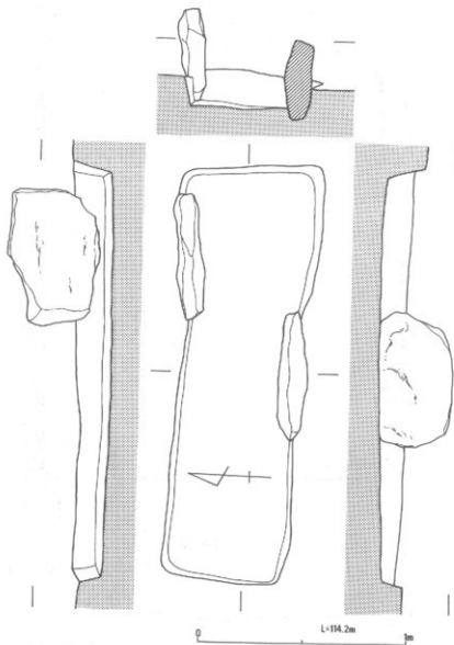
第13図 茶山2号墳中心主体図(S=1:40)
