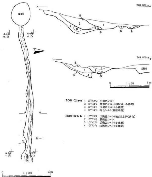
第18図 SD01・02溝
