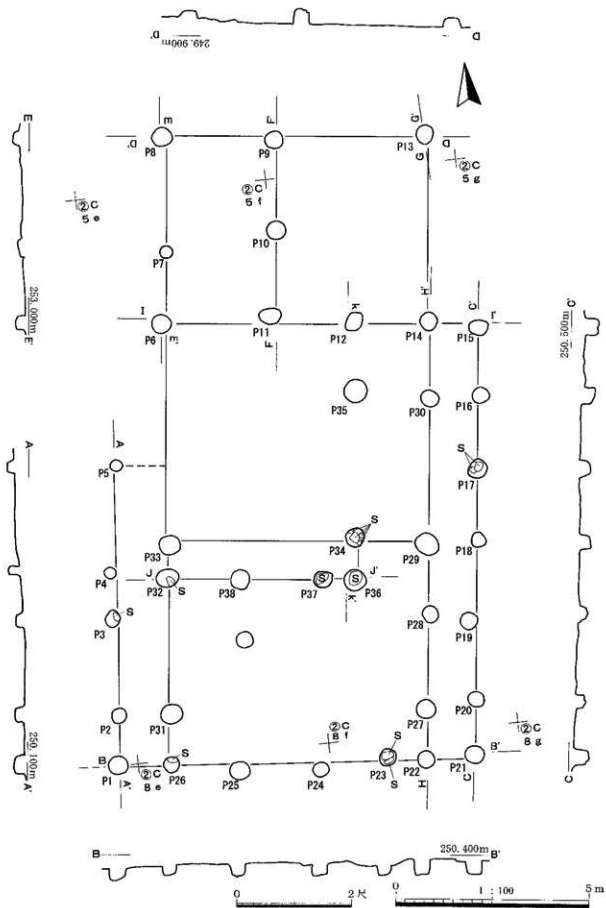
第10図 SB 01獨立柱建物
