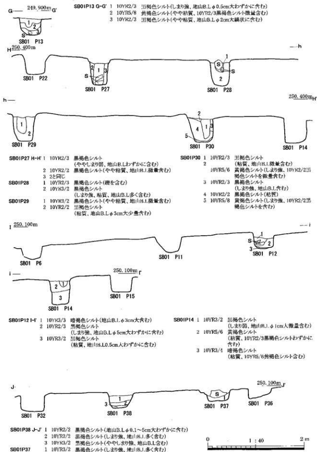
第13図 SB 01掘立柱建物断面(3)
