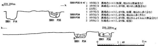
第14図 SB 01掘立柱建物断面(4)
