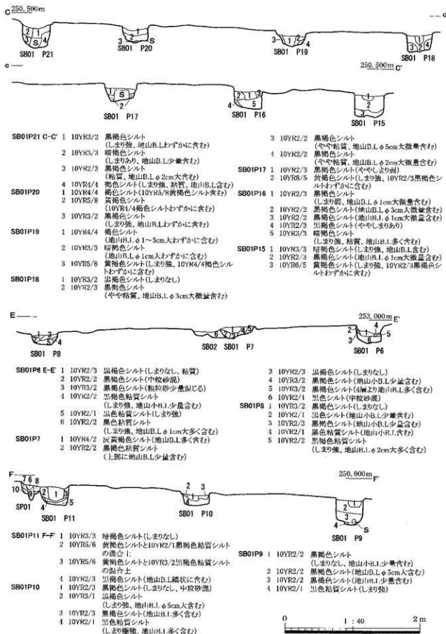
第12図 SB 01掘立柱建物断面(2)
