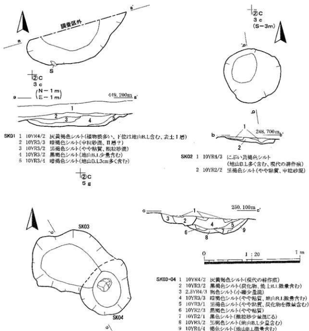
第16図 SK01~04土坑
