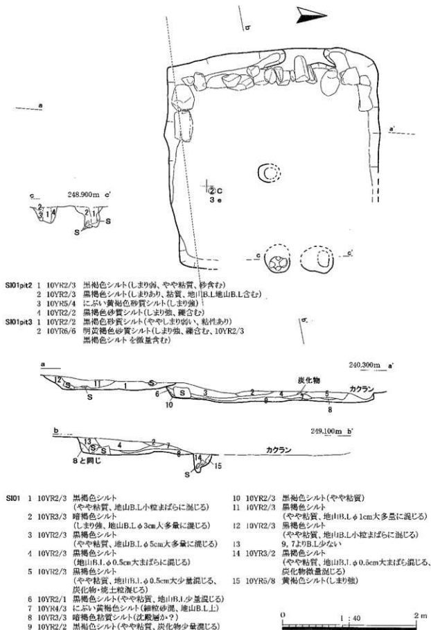
第7図 SI 01 竪穴住居
