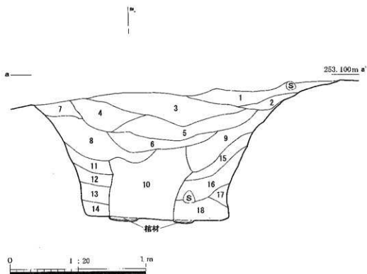
第30図 SZ09墓城
