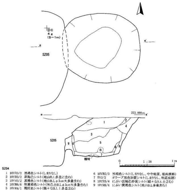
第25図 SZ04墓壇
