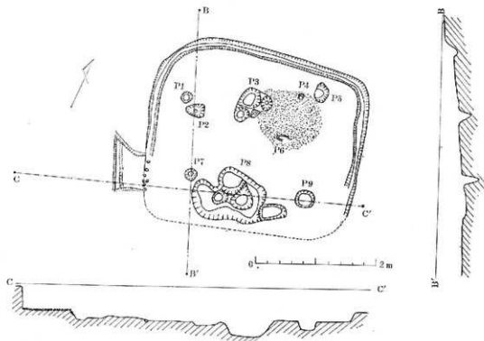
挿図第6 第6号住居址実測図
