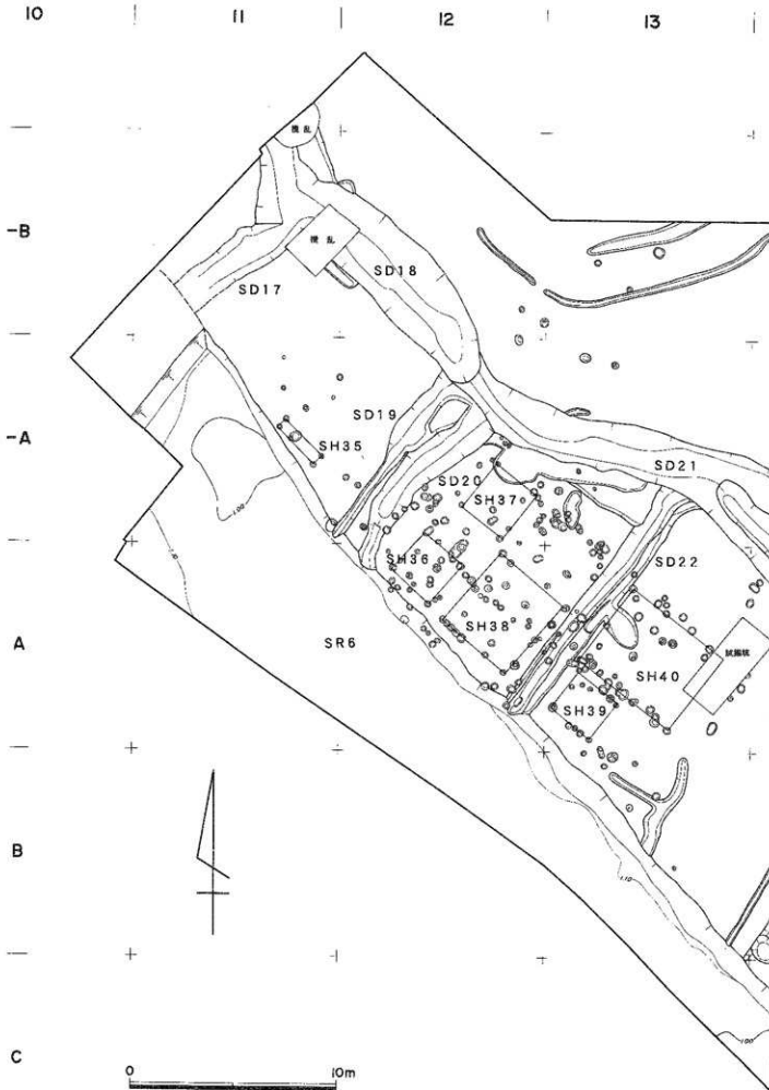
附圖4 10区第I遺構面全体圖
