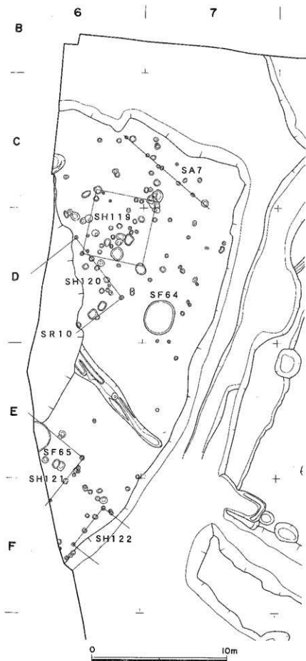
附图13 8区第IV遺構面全体図
