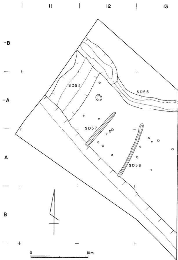
附图11 10区第Ⅲ层遗构面全体图
