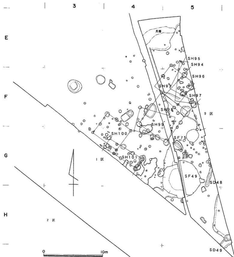
附圖5 1区・9区第II遺構面全体圖
