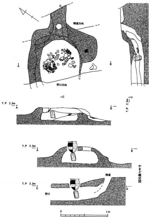
第4図 かまど平面及び断面図 (1/20)
