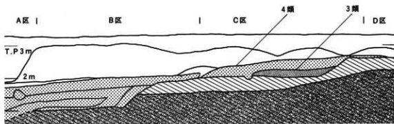
網目=平均満潮面 点線=平均干潮面 第6図 調査区1平面図及び横断模式図
