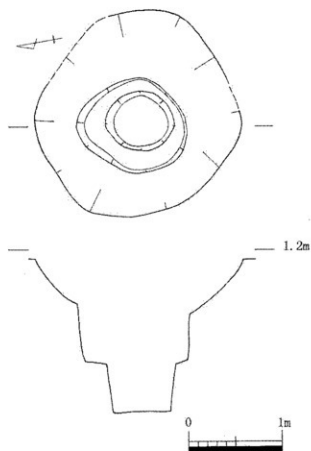
第13图 V区井戸4実測図
