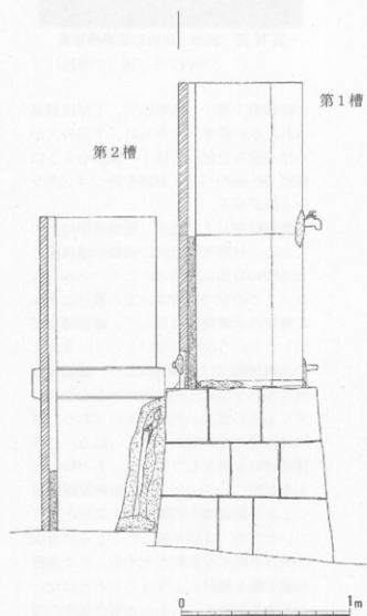
第13図 君津・銀座の濾過槽実測図(東から S=1/25)
