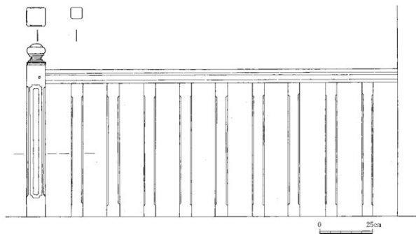
第15図 2階欄干実測図(西面)
