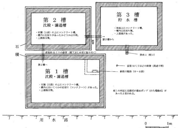
第 10 図 政津・土手根の濾過槽復元平面図（上が北 S=1/50）
