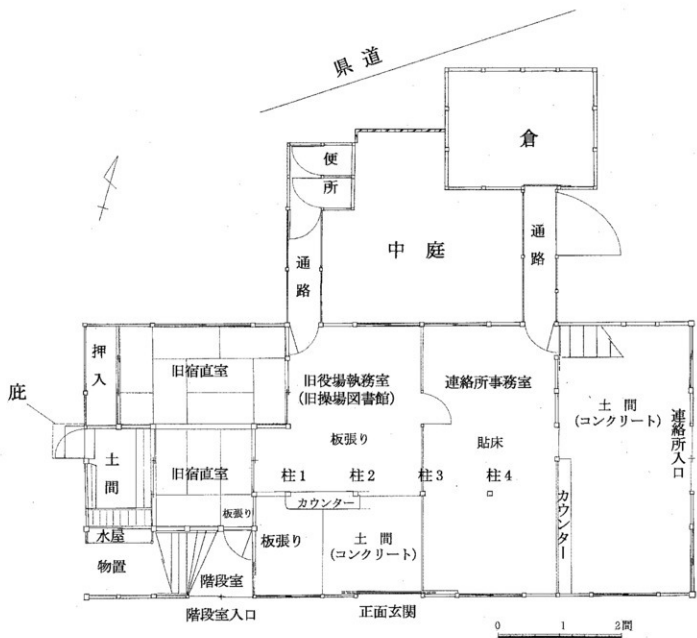
第8図 庁舎平面実測図 (上: 2階 下: 1階)
