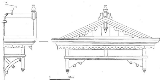
第9図 正面玄関庇実測図 (S=1/25)
