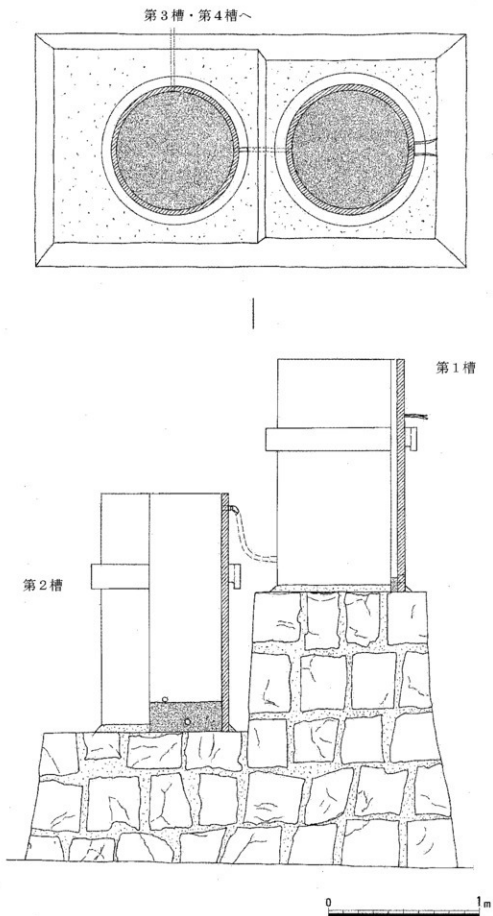
第8図 升田・横樋の濾過槽実測図（北からS=1/25） 図中表記は第11図参照
