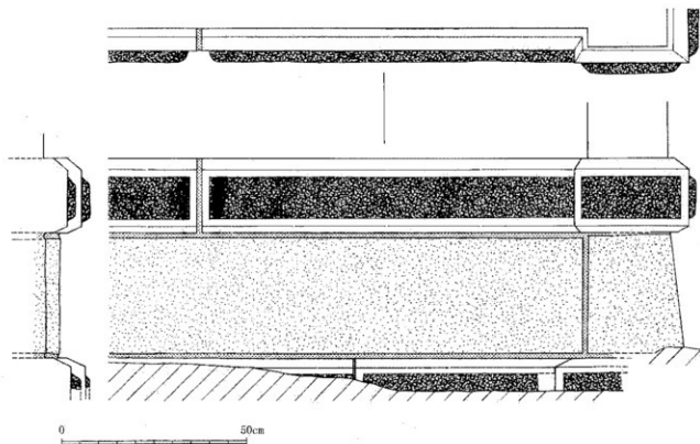
第17図 敷石実測図（建物南面東角部）
