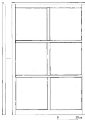
第 12 図 執務室の窓枠実測図
