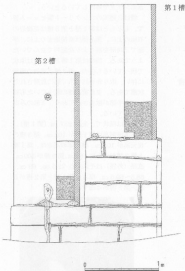
第11図 政津・川内の濾過槽実測図（南からS=1/25）
