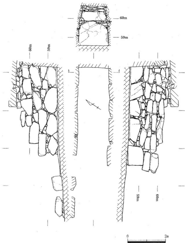
图3 横穴式石室实测图 (S=1/60)
