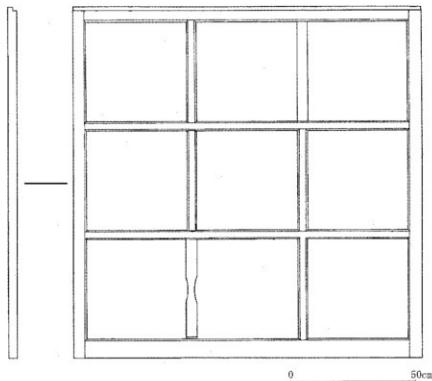
第 13 図 宿直室の窓枠実測図 (S=1/15 内側から)
