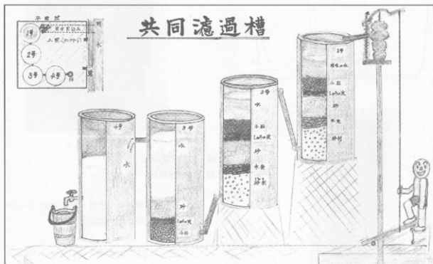
第6図「共同濾過槽」内部構成模式図（イラスト・岩崎徹堂氏）
