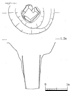
第15图 V区井戸511実測図
