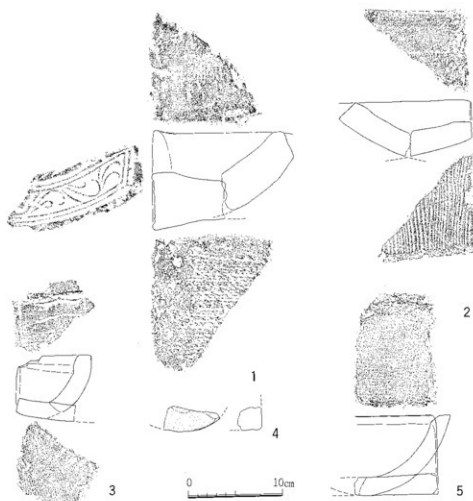
第5図 出土・採集瓦実測図
