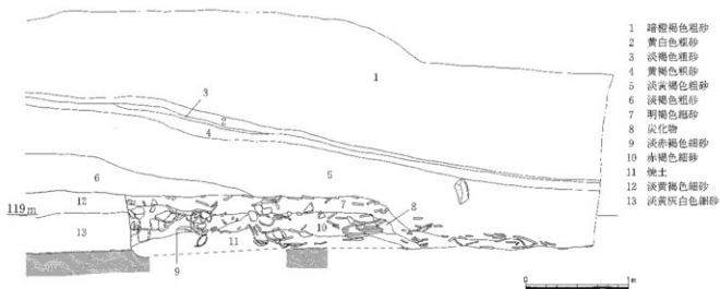
第9图 土层断面
