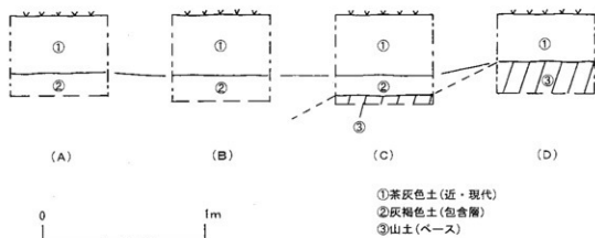
第4図 断面図
