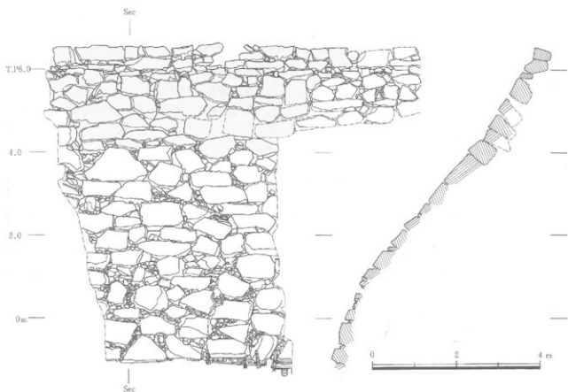
第8図 堀北岸高石垣立面・断面図 (S=1/80)
