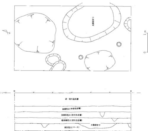
第4図 遺構図及び断面図
