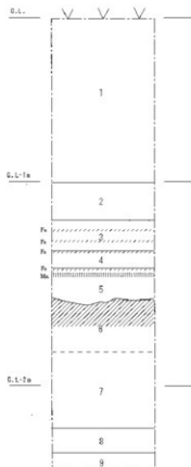
第2図 土層柱状図(1/20)
