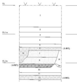
第2図 土層柱状図(1/20)
