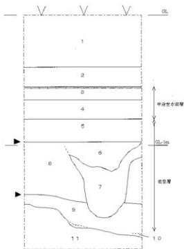
第2図 土層柱状図(1/20)
