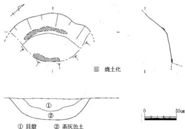
第7図 炉1
