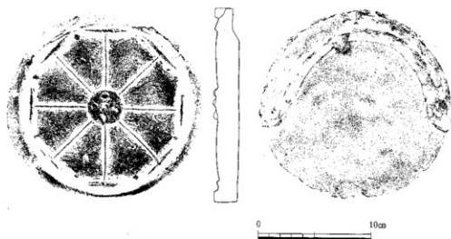
第6図 軒丸瓦
