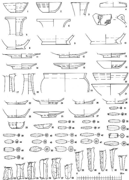
松崎貝塚Ⅰ区 10 層出土遺物実測図 2
