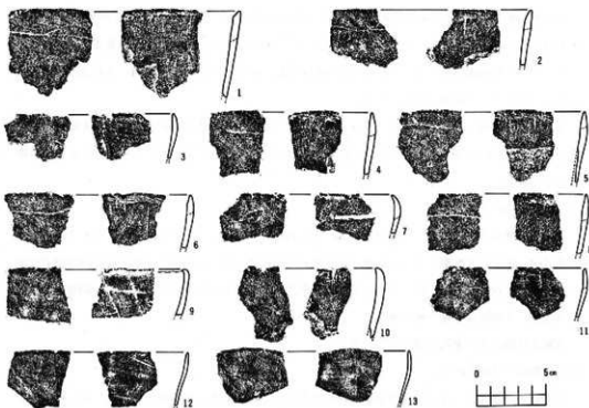
挿図6 製塩土器拓影(1~8=11層出土、9~11=6層出土、12=9層出土、13=Ⅱ区北貝層出土)
