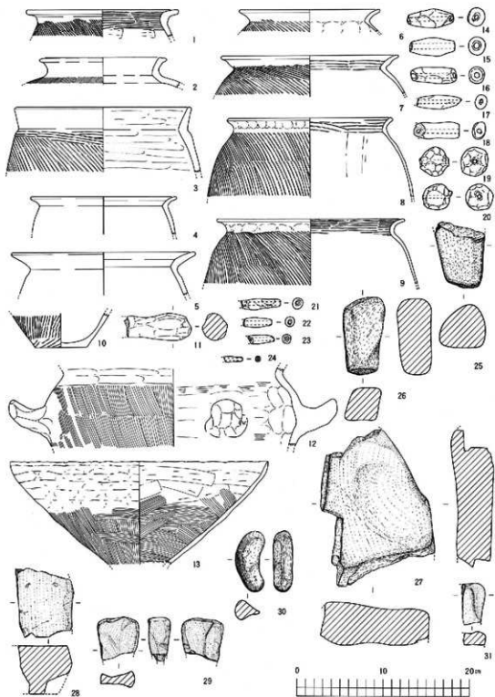
塚森遺跡出土土師器・土甕・石器実測図
