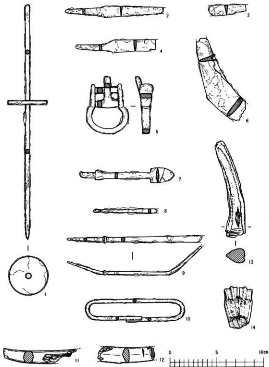
松嶋貝塚出土鉄器・骨角器実測図
