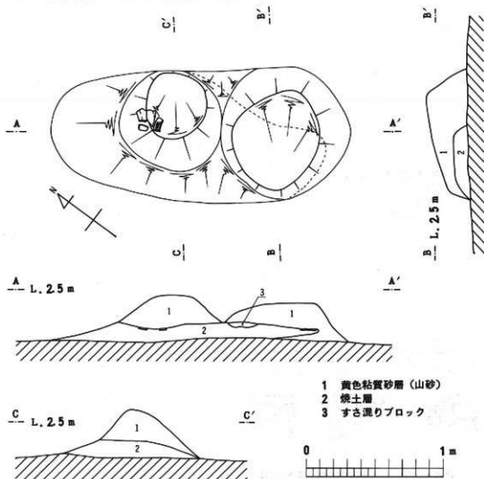
挿図3 Ⅴ-2遺構実測図
