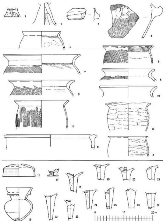
松崎貝塚 10 層出土および各所採集品実測図
