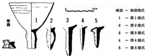
挿図9 知多式製塩土器の変遷
