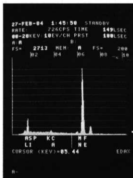
挿図 8 松崎貝塚Ⅱ区北貝層出土鉄塊およびEDAX特性X線チャート
