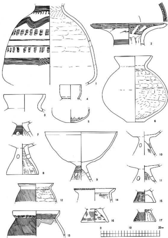
塚森遺跡出土弥生土器実測図
