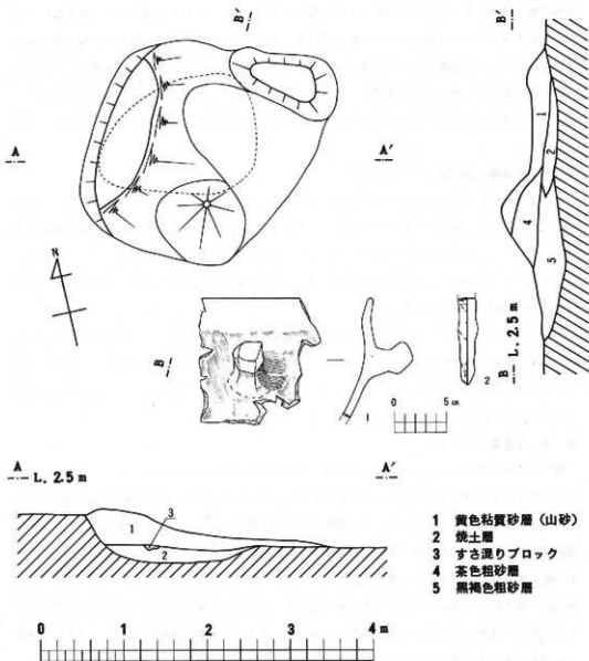
挿図2 Ⅱ-1遺構および出土遺物実測図
