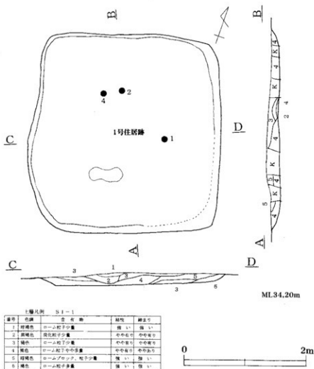
第3図 1号住居跡実測図
