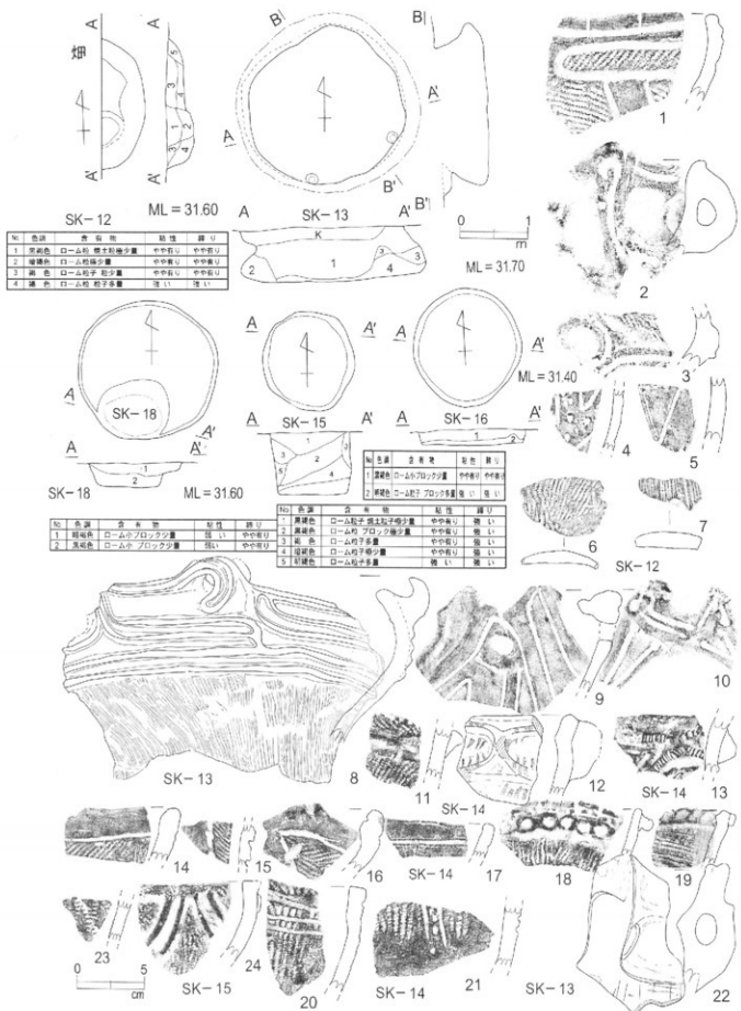
第9図 SK-12、13、14、15、16号遺構と出土遺物実測図
