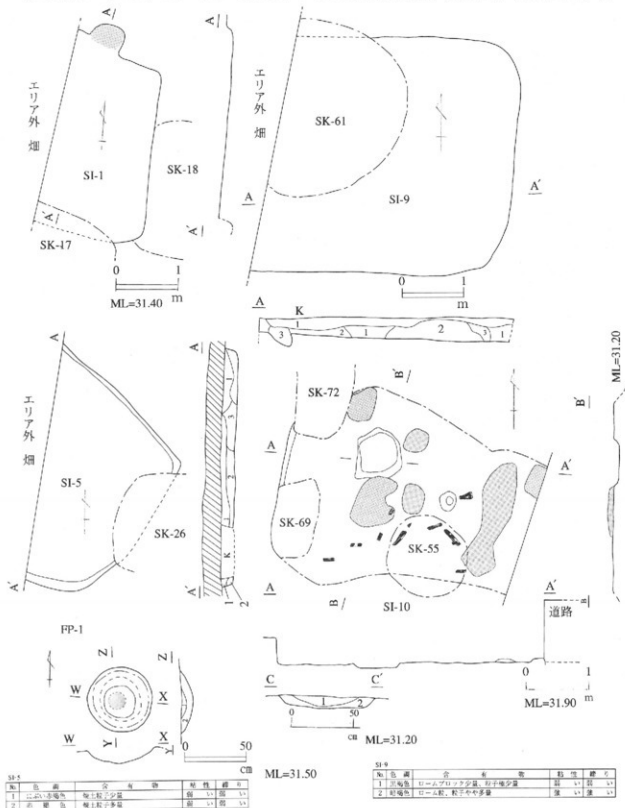
第4図 第1・5・9・10号住居跡、F P-1実測図
