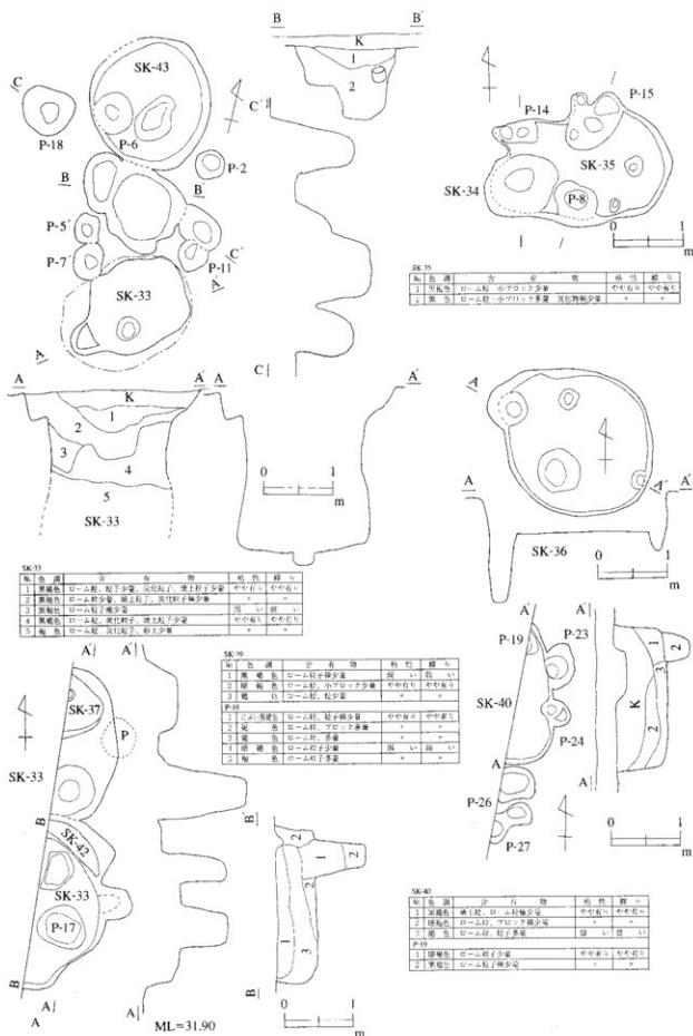
第18图SK-29'、32、33、34、35、36、37、38、39、40、42、43号実測図
