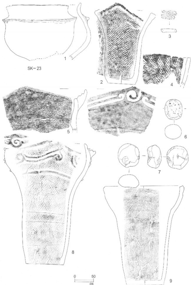
第14图 SK-23号出土遗物实测图
