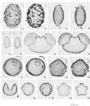
図版1 寄生虫卵・花粉化石(1)
