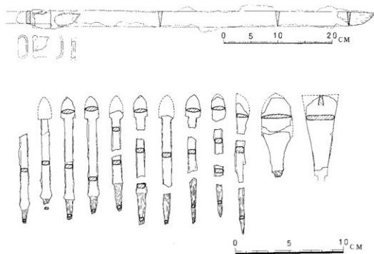
第8図 石室出土武器類実測図
