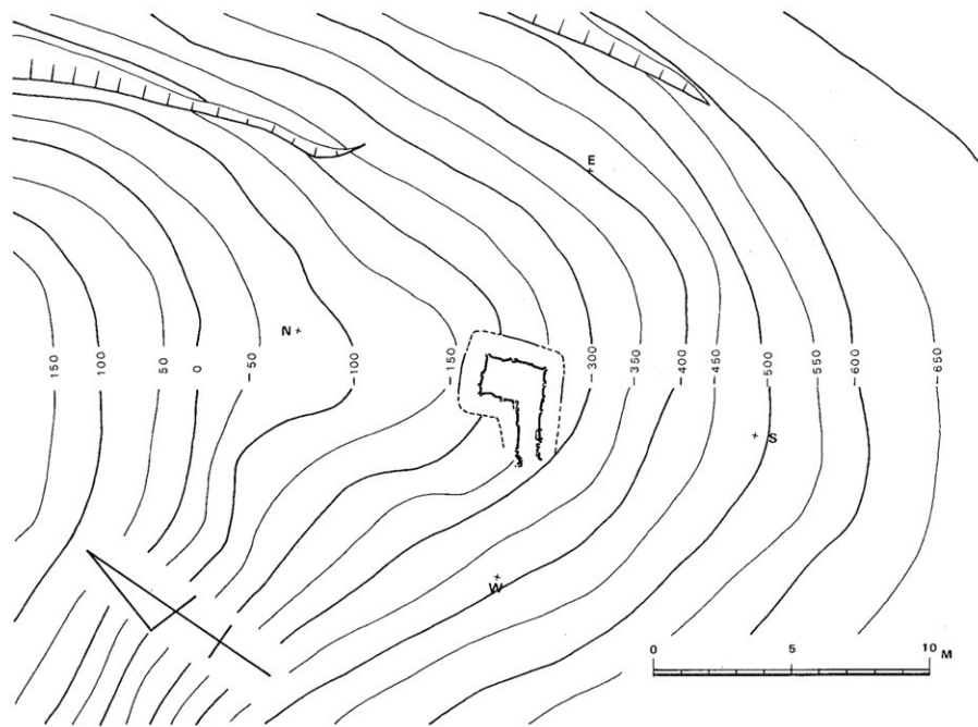
墳丘実測図
