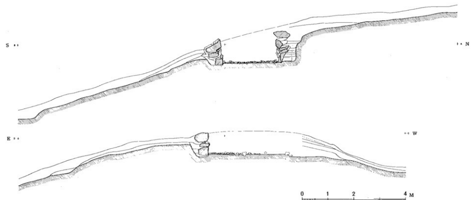
墳丘実測図
