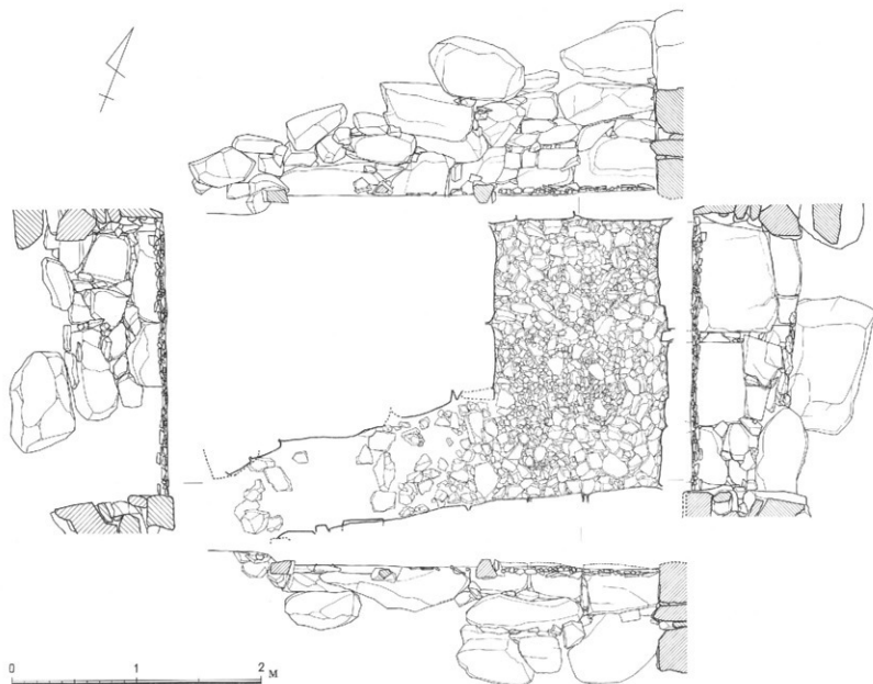
石室実測図
