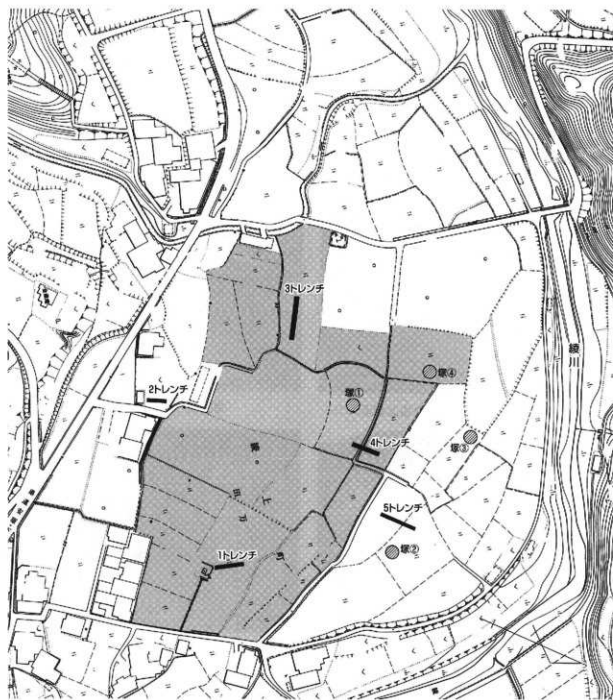
第43図 トレンチ配置図 (S=1/2,000) ■■■■■…出晴遺跡範囲
