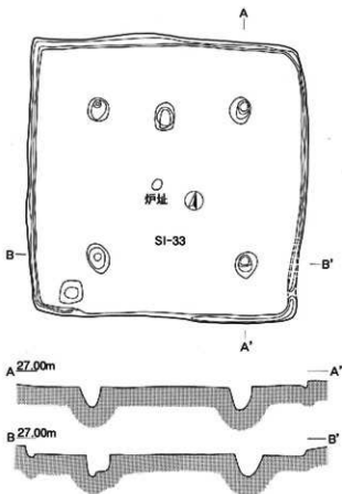
第33号住居跡 (SI-33) 実測図
