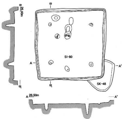
第80号住居跡, 第48号土坑 (SI-80, SK-48) 実測図
