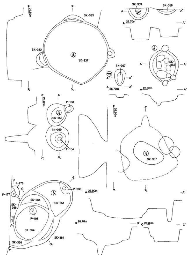
第161図 御天遺跡土坑実測図10 (SK-337・351・352・353・354・357・358・359・360・364・366・367・368・382・383, S=1:50)
