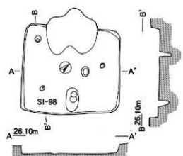
第98号住居跡 (SI-98) 実測図
