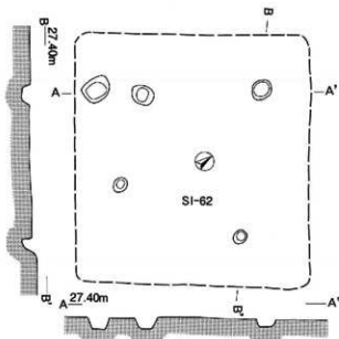
第62号住居跡 (SI-62) 実測図
