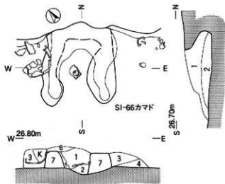
第66号住 (SI-66) カマド
