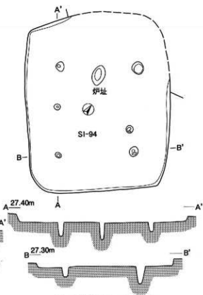
第94号住居跡 (SI-94) 実測図
