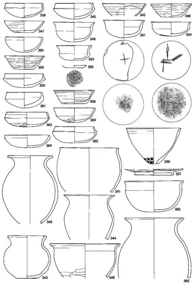
第187図 初賀場遺跡出土遺物実測図12 (No.338~365, S=1:4)
