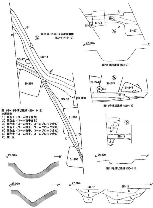
第136図 初買場遺跡溝状遺構実測図2 (平面図S=1:250, S.L., E.L.S=1:60)
