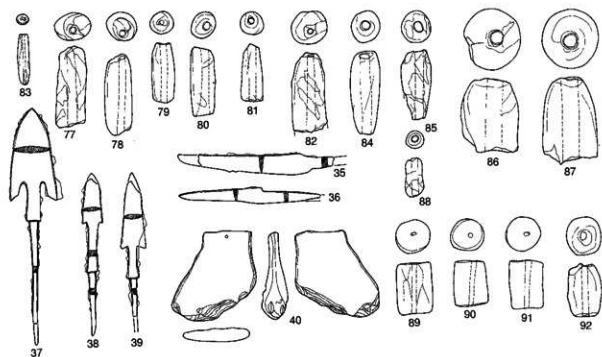
第227图 木田余台遺跡群出土遺物実測図4 (No.37~40, 鉄製品・No.77~92, 土製品・石製品, S=1:3)
