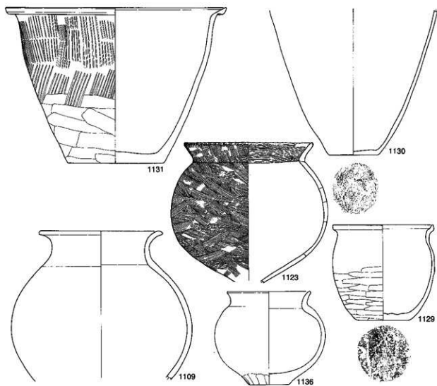
第220圖 宝積遺跡出土遺物実測図6 (No.1109~1136, S=1:4)
