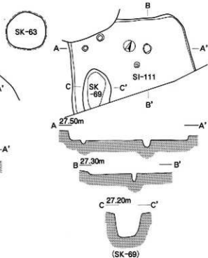
第111号住居跡, 第69号土坑 (SI-111, SK-69) 実測図
