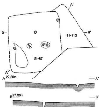
第87号・112号住居跡 (SI-87・112) 実測図
