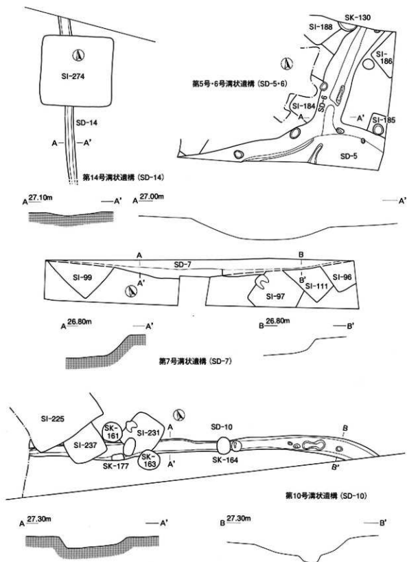
第138图 初買場遺跡溝状遺構実測图4 (平面图S=1:250, E.L.S=1:50)
