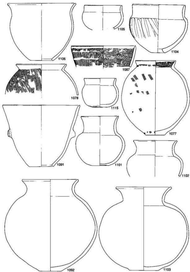
第 217 图 宝積遺跡出土遺物実測図 3 (No.1077~1115, S=1:4)
