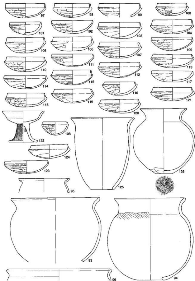
第179図 初買場遺跡出土遺物実測図4 (No.93~126, S=1:4)
