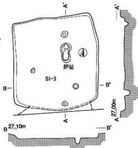
第3号住居跡 (SI-3) 実測図
