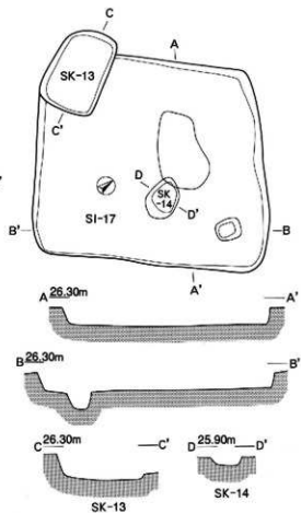
第17号住居跡, 第13号・14号土坑 (SI-17, SK-13・14) 実測図
