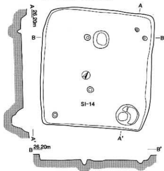
第14号住居跡 (SI-14) 実測図
