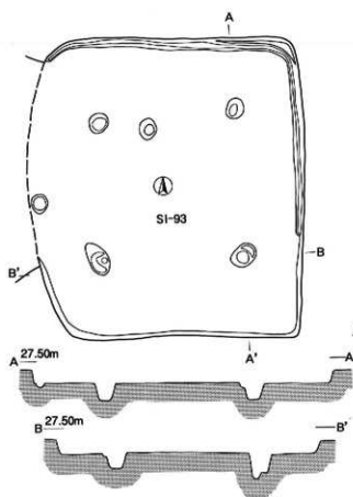
第93号住居跡 (SI-93) 実測図
