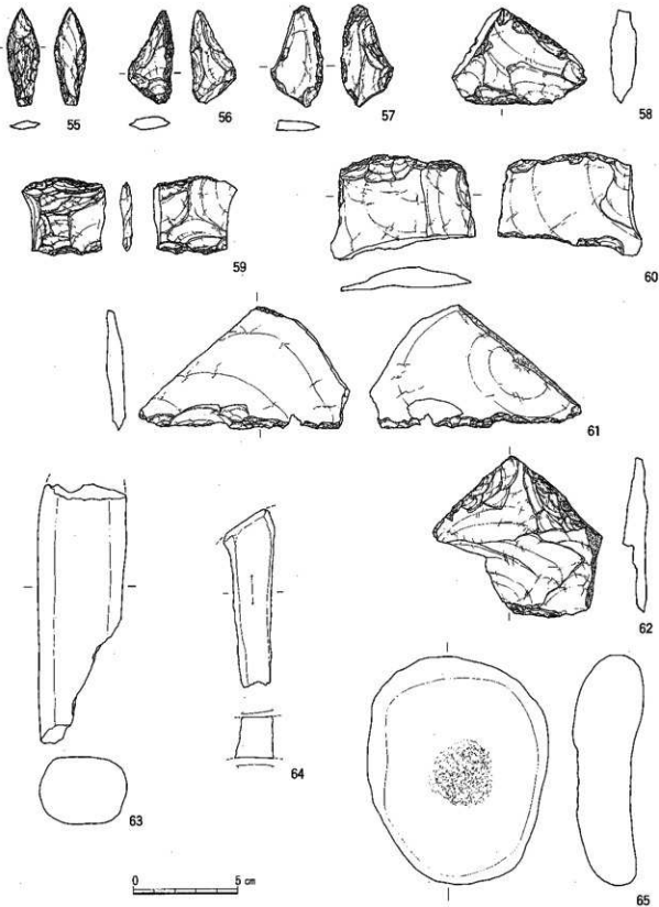
第17图 SH-01 出土石器实测图
