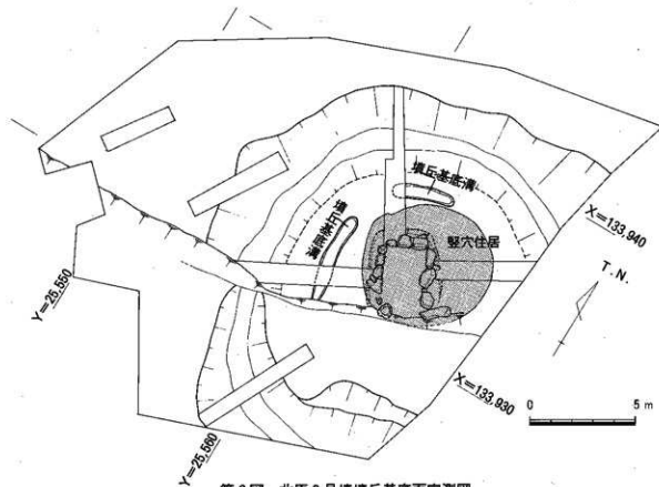
第6図 北原3号墳墳丘基底面実測図
