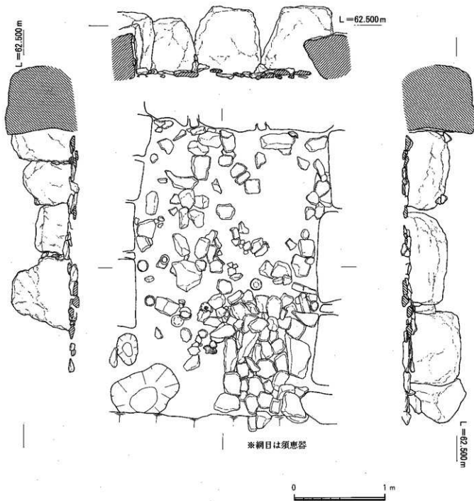
第8図 北原3号墳石室実測図
