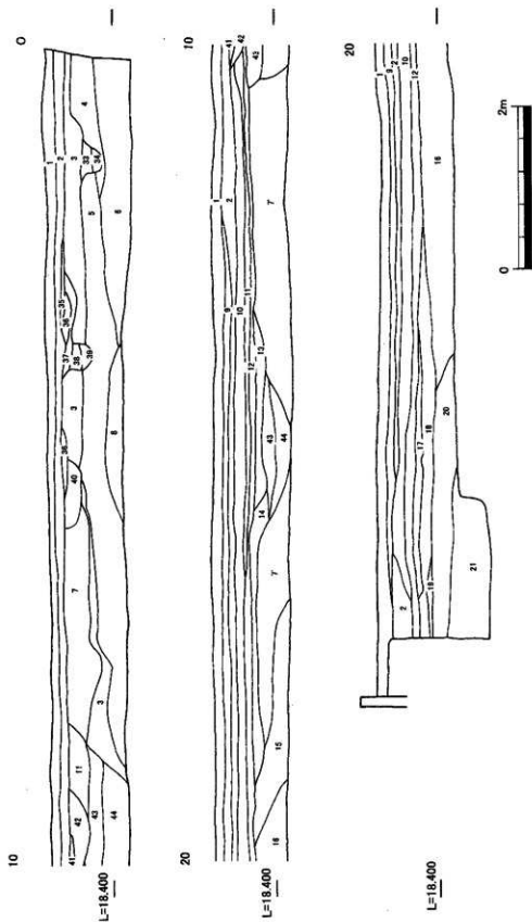
第10図 A調査区第1トレンチ基本土層図
