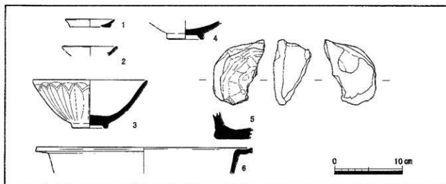
第34図 SE01出土遺物実測図
