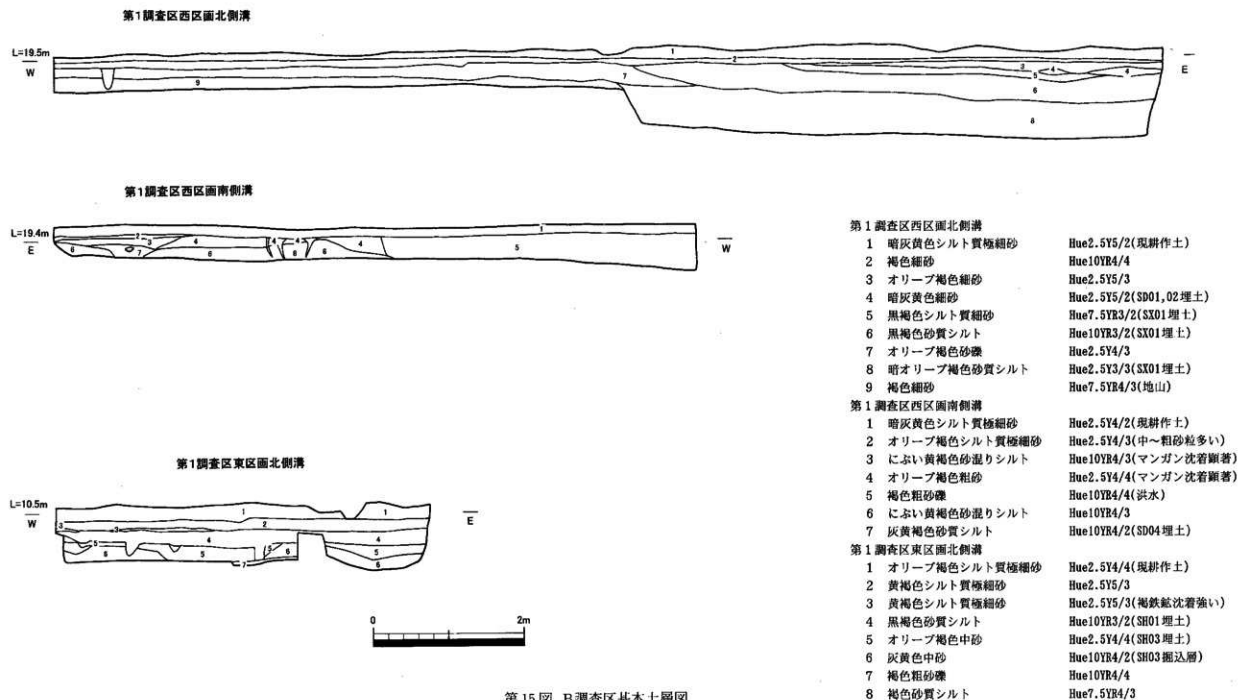
第15図 B調査区基本土層図
