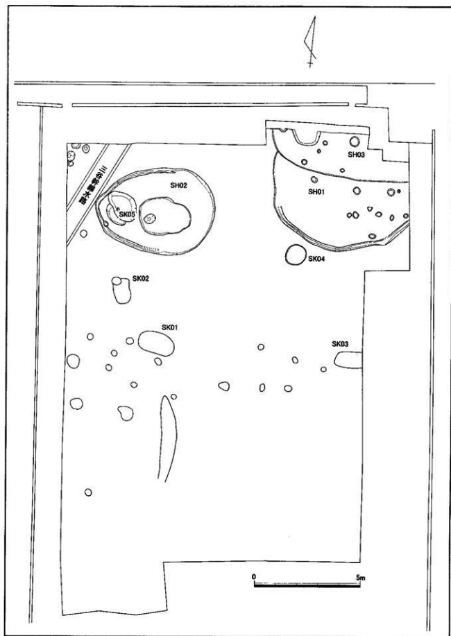
第28図 B調査区東区画遺構配置図
