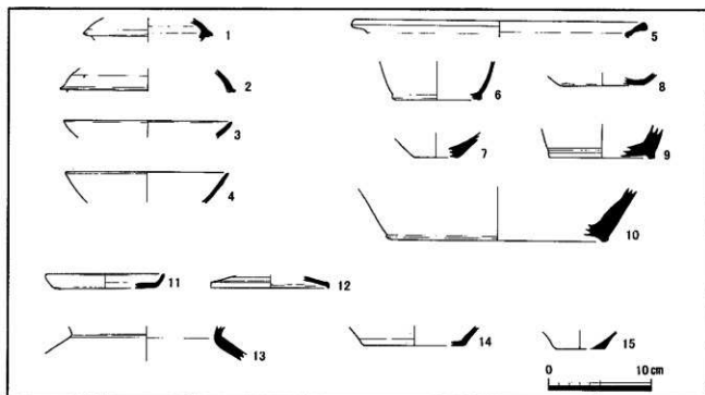
第73図 南海道推定地第3調査区出土遺物実測図
