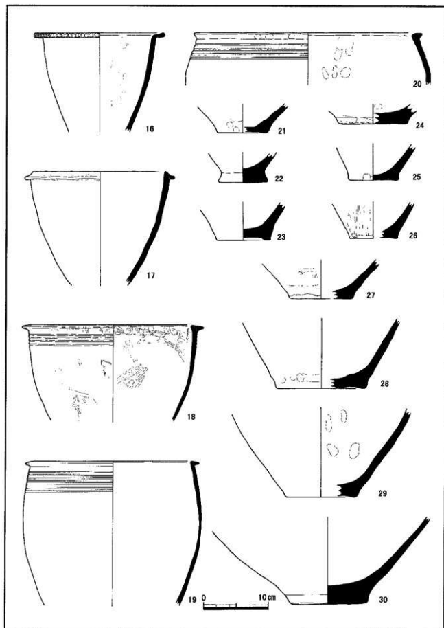
第58図 F調査区SD01第2トレンチ出土遺物実測図②
