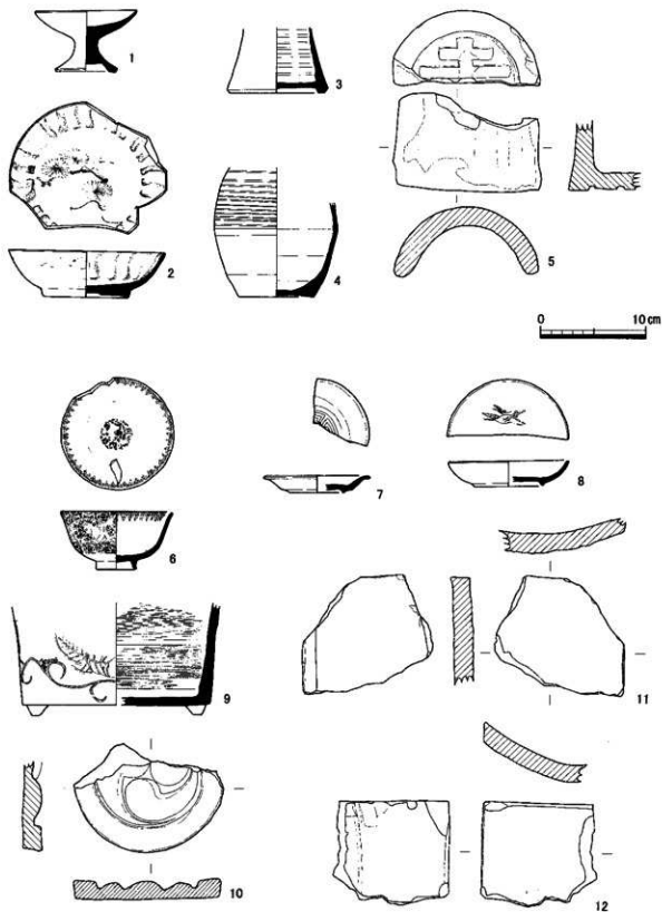
第25図 C調査区SD05出土遺物実測図
