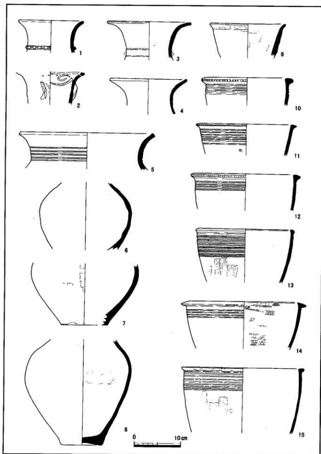
第57図 F調査区SD01第2トレンチ出土遺物実測図①
