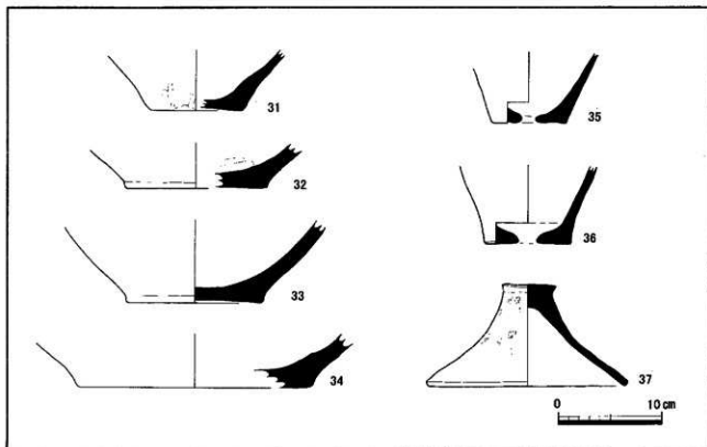
第59図 F調査区SD01第2トレンチ出土遺物実測図③
