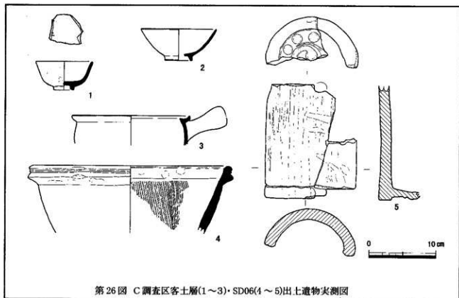
第26図 C調査区客土層(1～3)・SD06(4～5)出土遺物実測図
