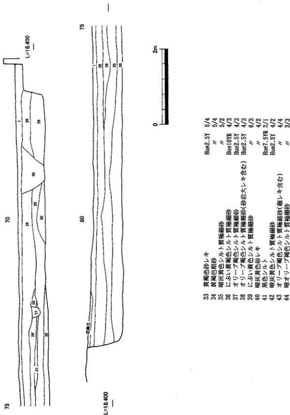
第13図 A調査区第4トレンチ基本土層図
