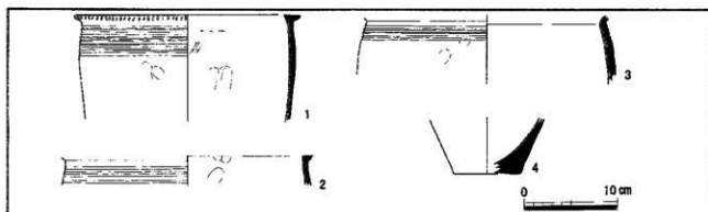
第44図 SK01(西)出土遺物実測図
