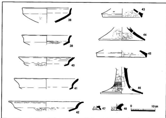
第79図 田園北地区SD02出土遺物実測図③
