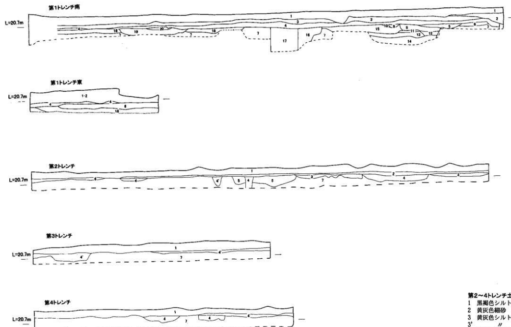
第20図 F調査区基本土層図
