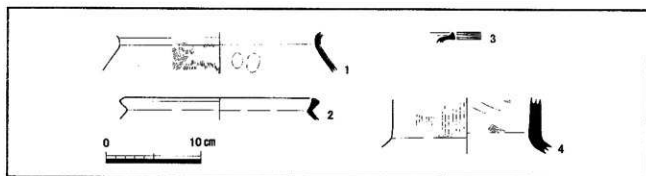
第38図 SH01出土遺物実測図
