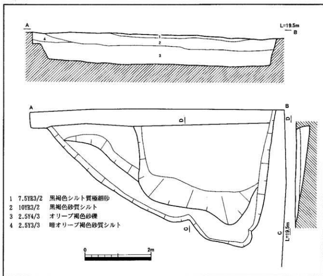
第35図 SX01遺構図・土層断面図
