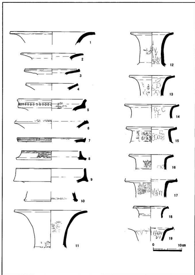
第80図 田岡北地区SD02下層出土遺物実測図①
