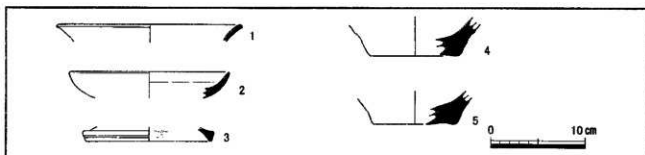
第40図 SH02出土遺物実測図
