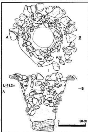
第33図 SE01遺構図
