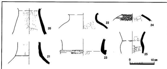
第81図 田岡北地区SD02下層出土遺物実測図②
