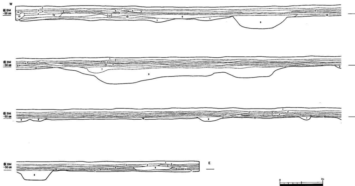
第17図 E調査区第1トレンチ基本土層図
