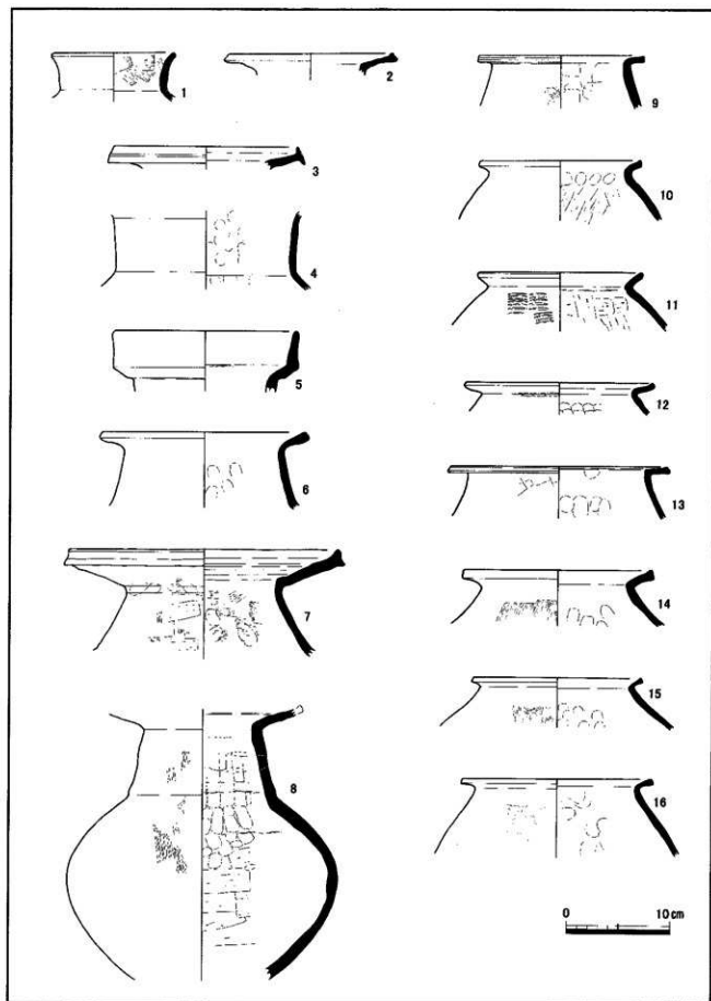
第77図 田岡北地区SD02出土遺物実測図①
