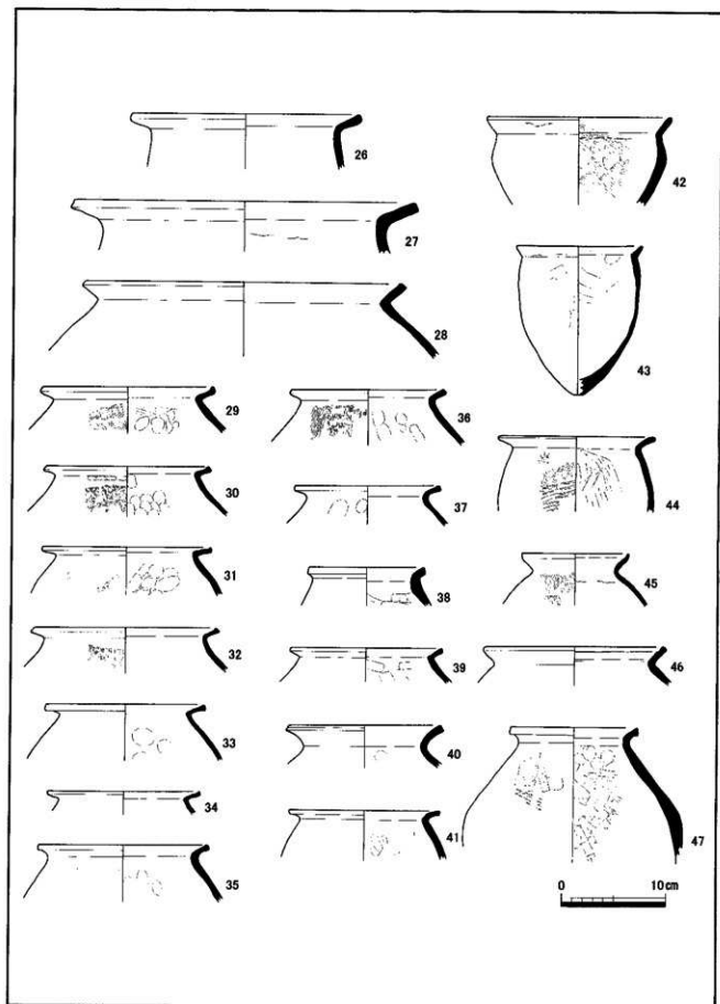
第82図 田国北地区SD02下層出土遺物実測図③
