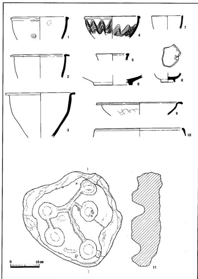
第60图 F调查区SD03石组中出土遗物实测图①
