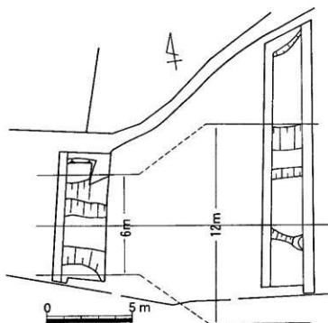
第12図 南海道幅員想定図
