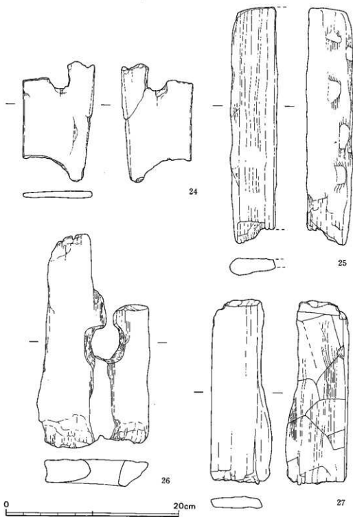
Fig 7. 木器実測図 5 板状木製品
