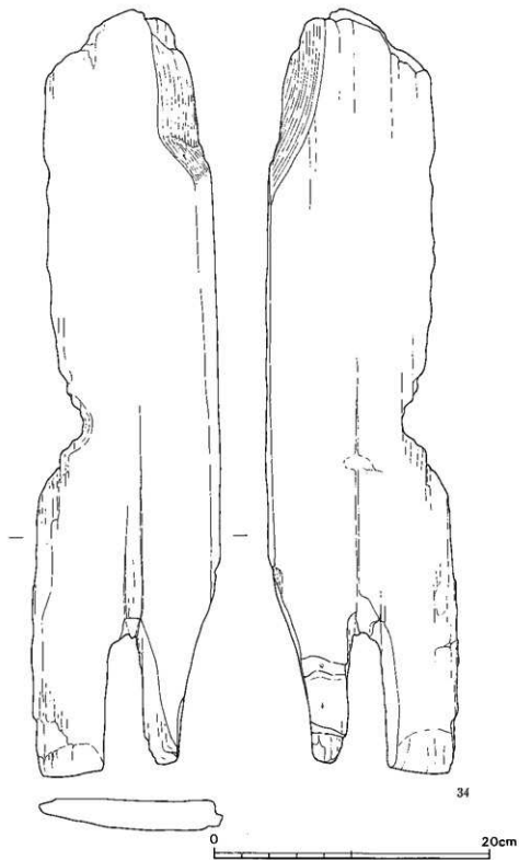
Fig 9. 木器実測図 7 板状木製品
