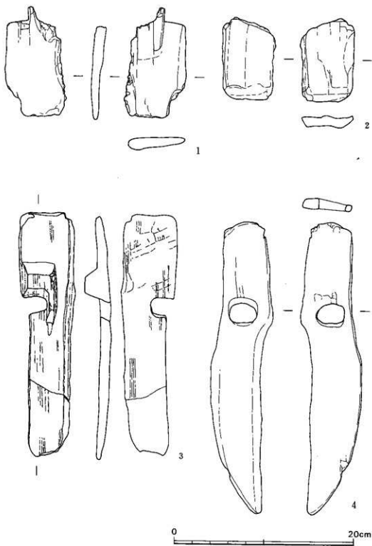
Fig 3. 木器実測図 1 器(1~4)
